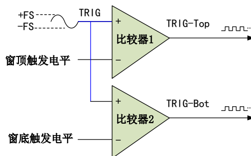
图5-3-4 比较器
