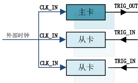
图 4-9-2 采用共同外时钟
