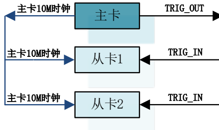
图 4-9-1 主从卡级联
