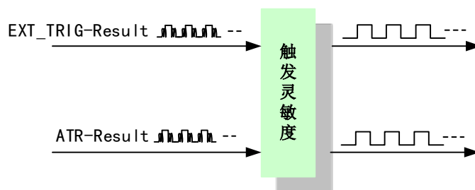
图 5-1-2 触发灵敏度
