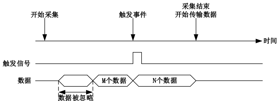
图 4-8-2-2 中间触发
