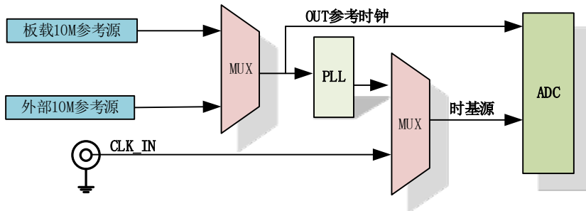
图 4-7-1 时基源框图
