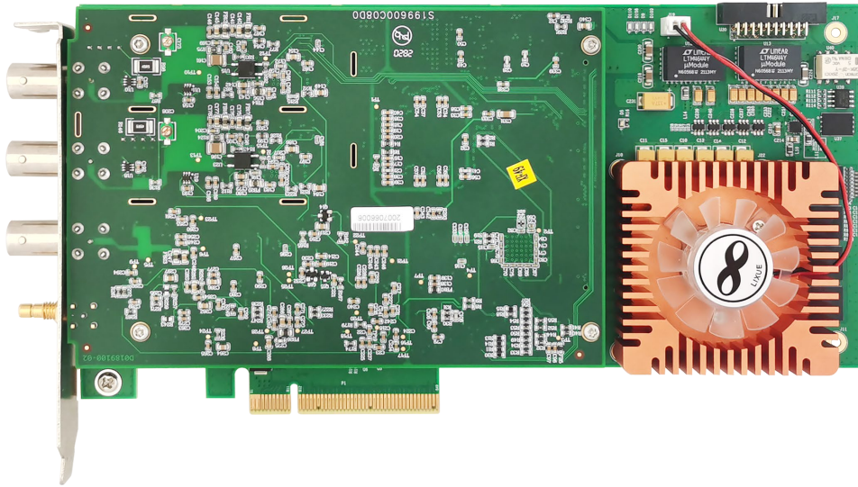
图 3-3-1 PCIe8910M 产品外观图
