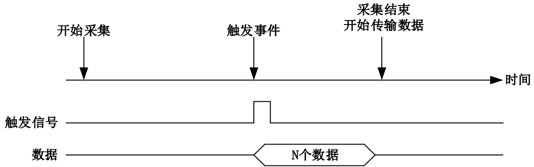
图 4-8-2-3 后触发
