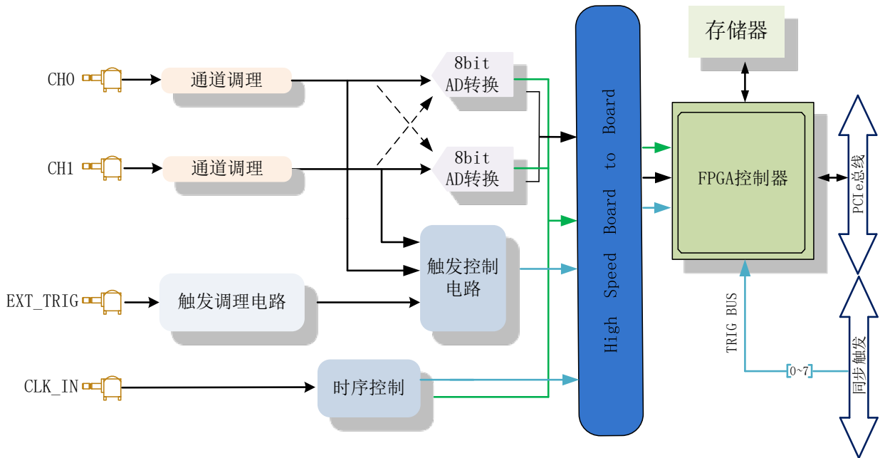
图 3-1-1 PCIe8910M 系统框图
