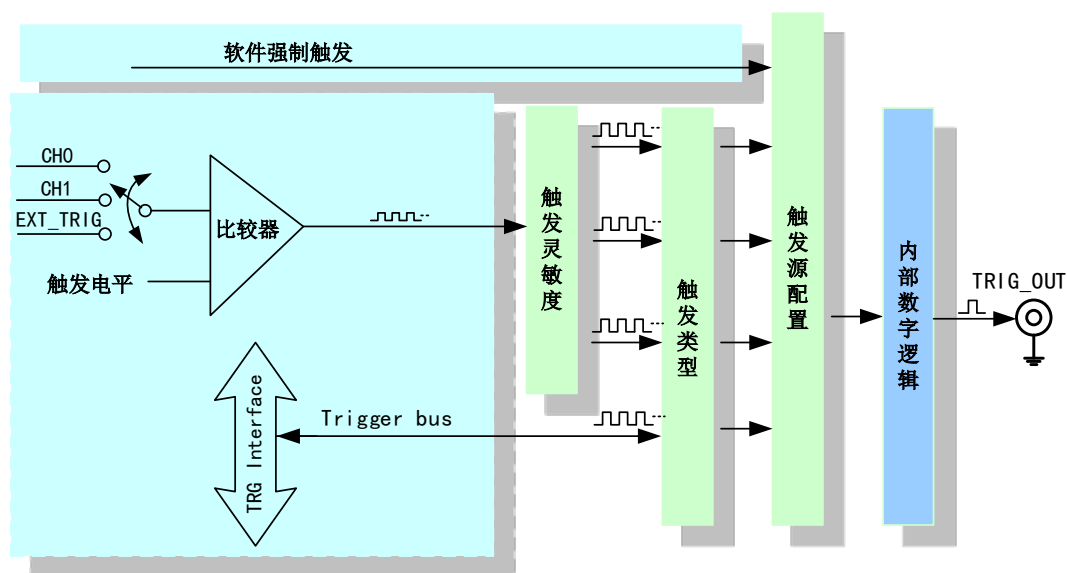
图 5-1-1 AD 触发功能框图
