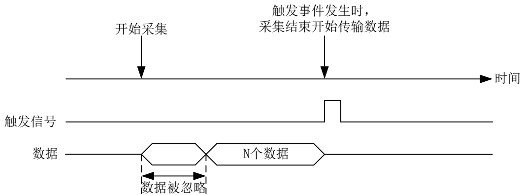
图 4-8-2-4 预触发
