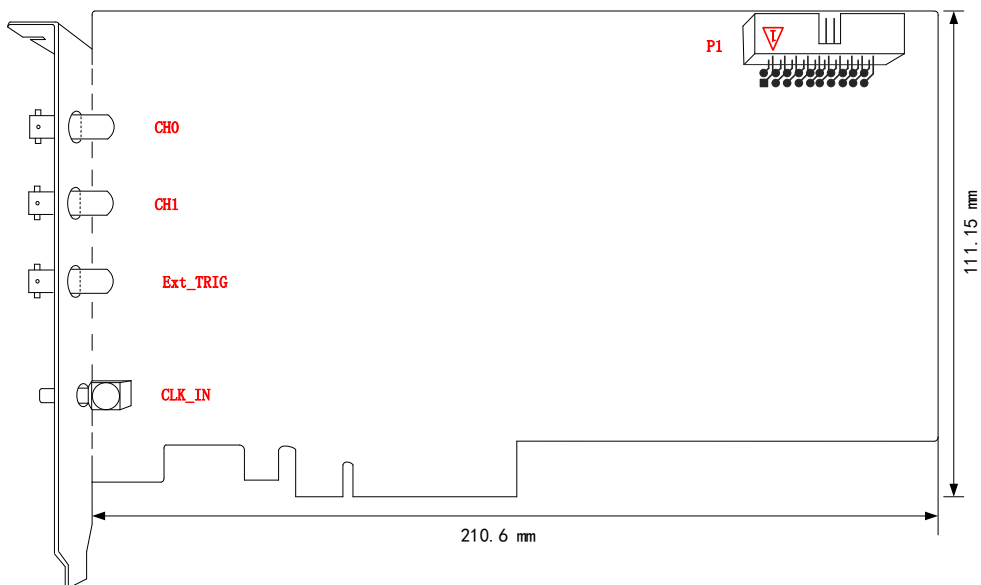
图 3-2-1 PCIe8910M 板卡尺寸图
