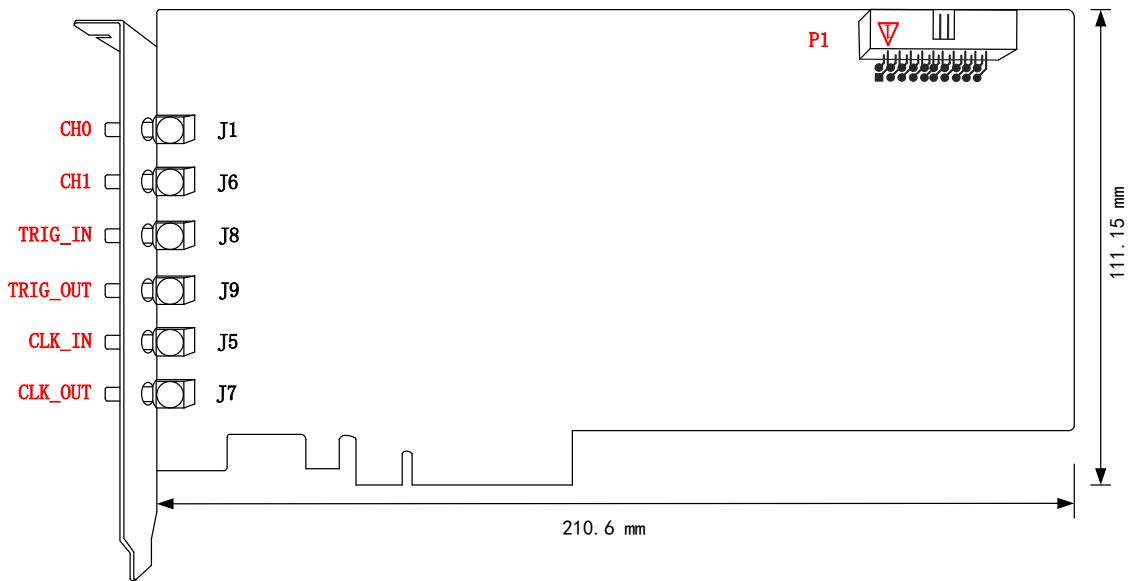
图 3-2-1 PCIe8922M 板卡尺寸图
