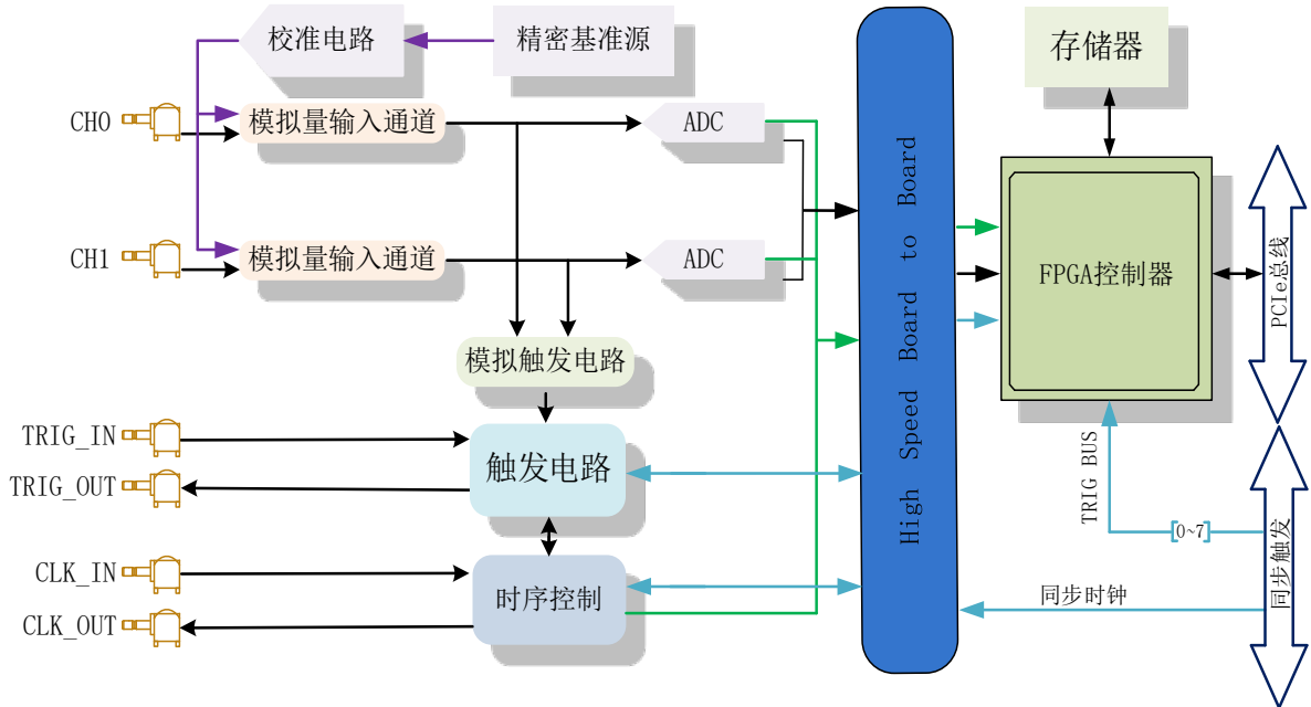
图 3-1-1 PCIe8922M 系统框图
