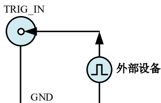
图 4-8-7 DTR 触发信号连接
