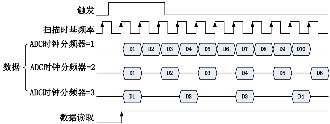
图 4-7-2 AD 抽样速率示意图
