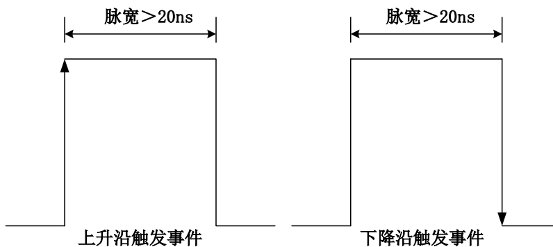
图 4-8-8 脉宽最小值图
