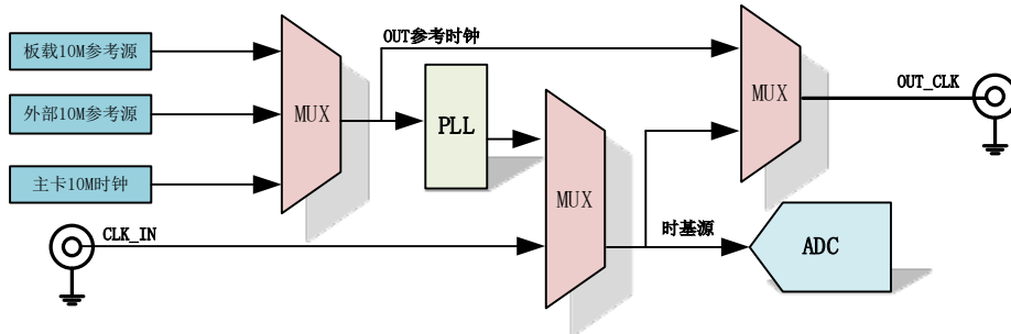
图 4-7-1 时基源框图
