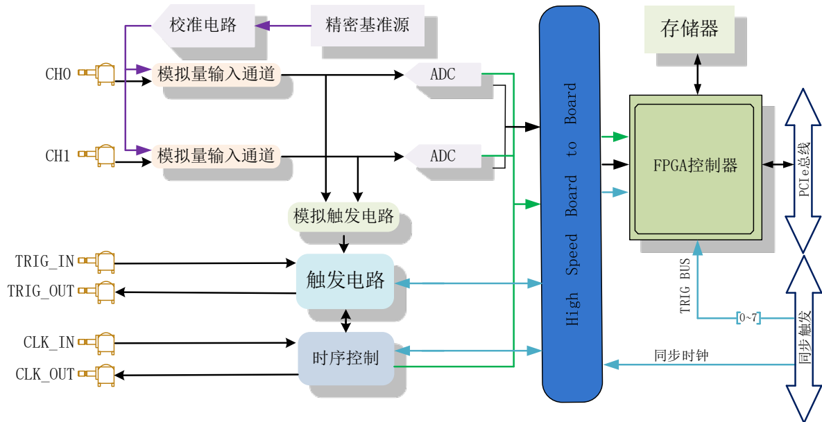
图 3-1-1 PCIe891xM 系统框图
