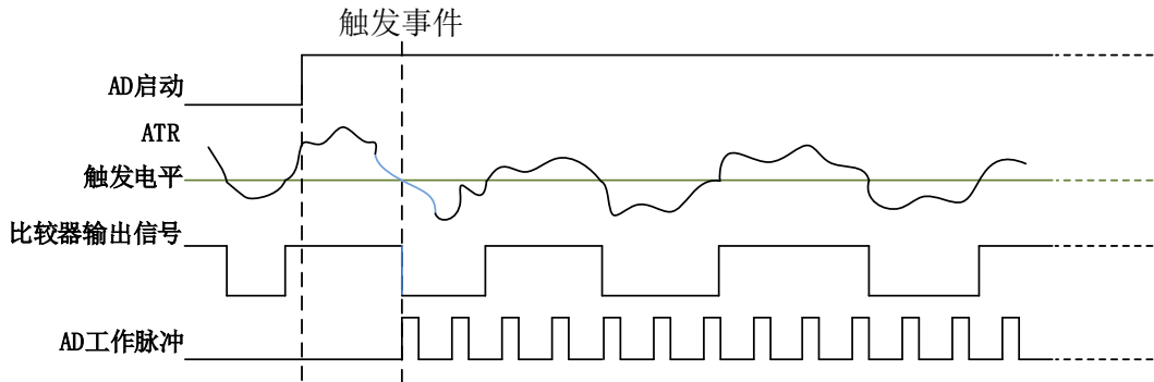
图 4-8-6 ATR 触发--下降沿触发
