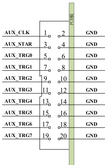
图 3-4-1 P1 管脚定义
