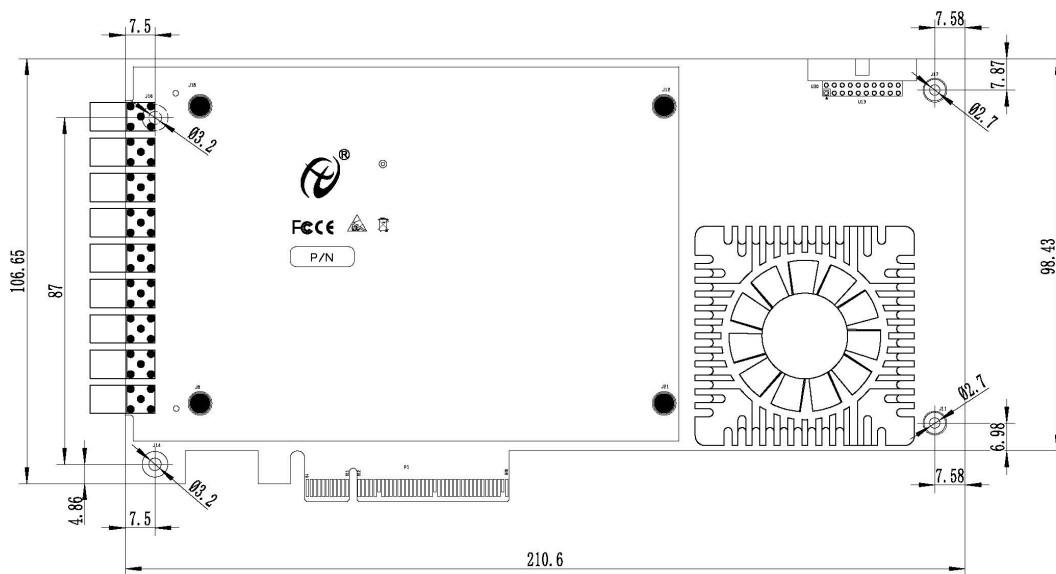
图 3-2-1 PCIe858xM 板卡尺寸图
