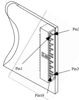
图 3-3-3 RTSI 的 Pinout 图
