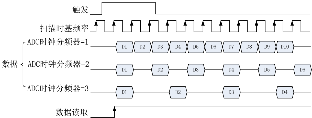
图 4-7-2 AI 抽样速率示意图
