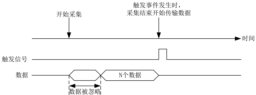
图 4-10-4 预触发
