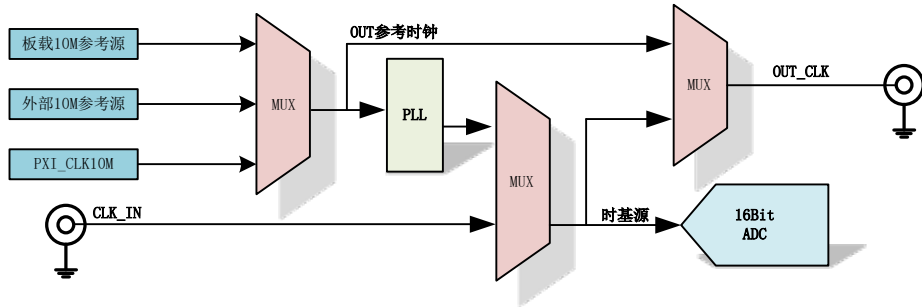
图 4-7-1 时基源框图
