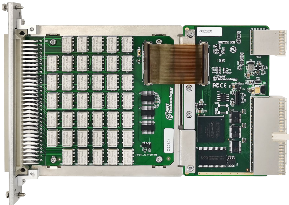
图 3-1-1 PXI2604 外形图
