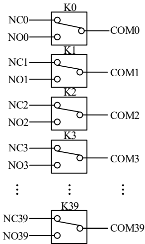
图 2-2-1 硬件框图
