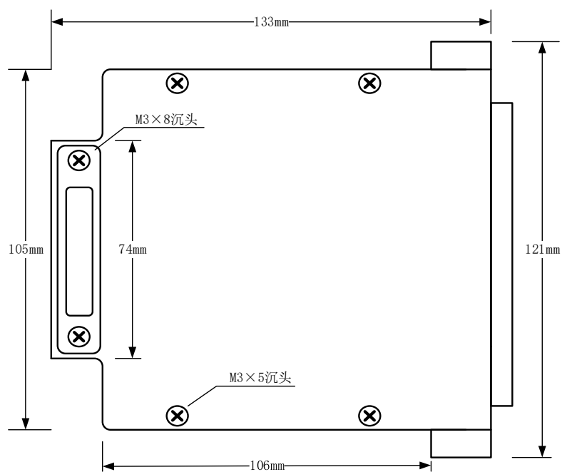
图 3-1-3 TB2604 尺寸图
