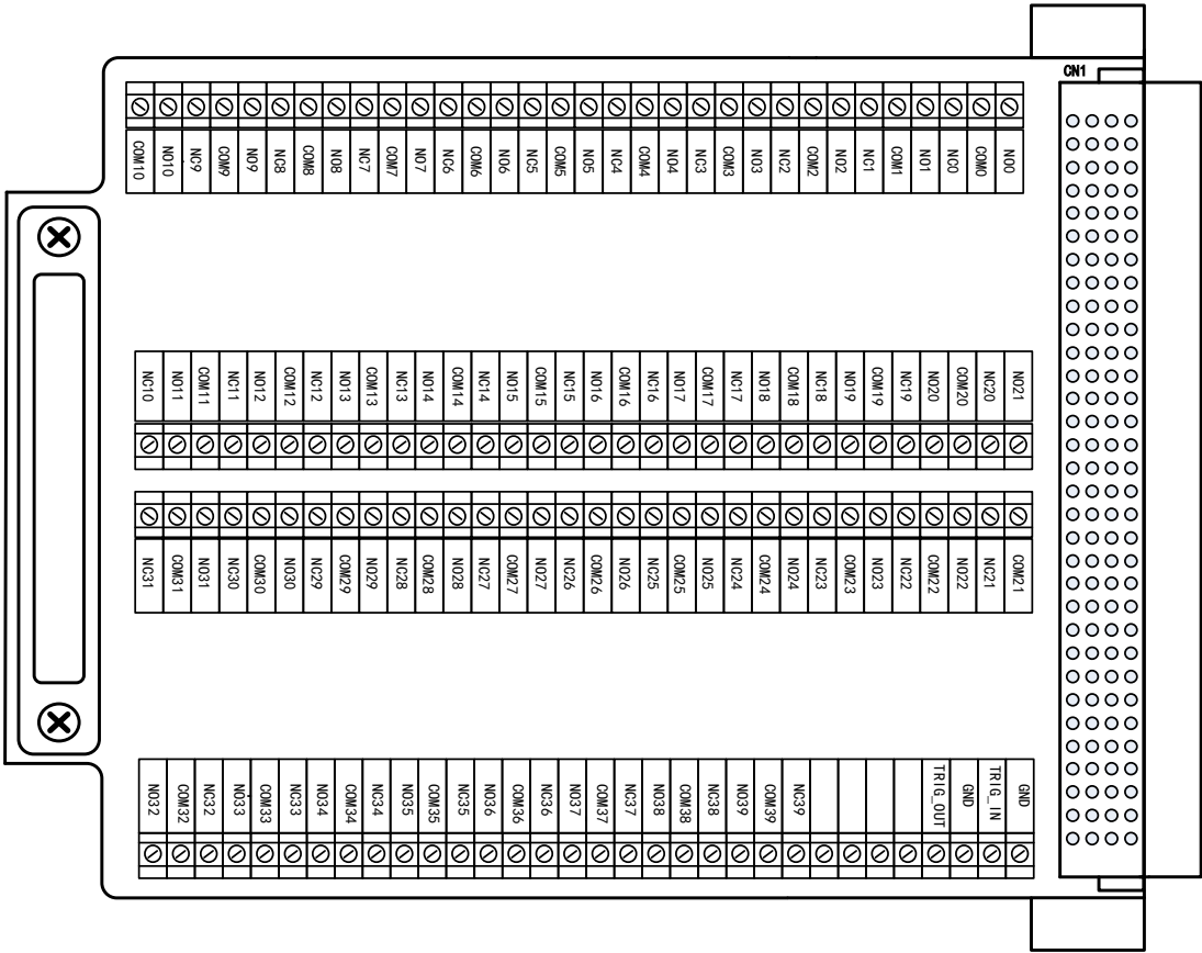
图 3-3-1 TB2604 端子盒接线定义图
