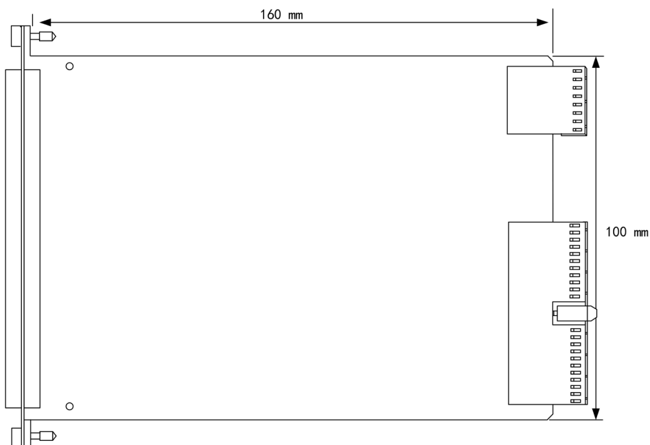
图 3-1-2 PXI2604 尺寸图
