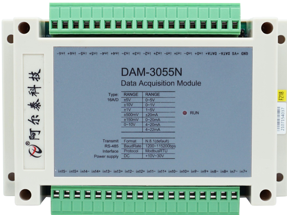
图 2 V6.03 以后版本，两侧端子为插拔式接线端子
