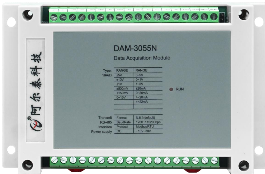
图 1 V6.02 以前版本，两侧端子为螺钉式接线端子
