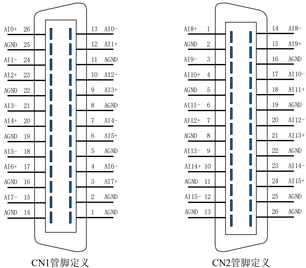
图 3-3-1 PCI8815 连接器定义图
