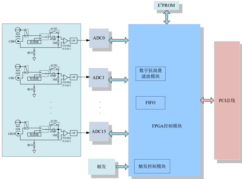
图 2.2.1 PCI8815 系统框图
