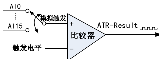
图4-8-7 比较器
