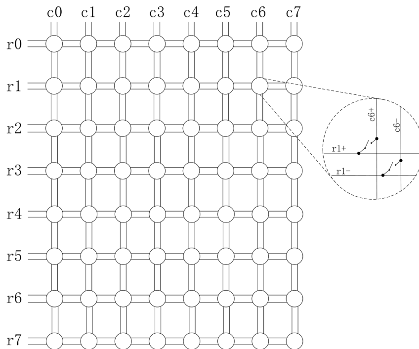
图 2-2-2 2 线 8 \times 8 矩阵
