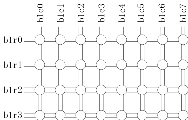
图 2-2-3 2 线双 4 \times 8 矩阵
