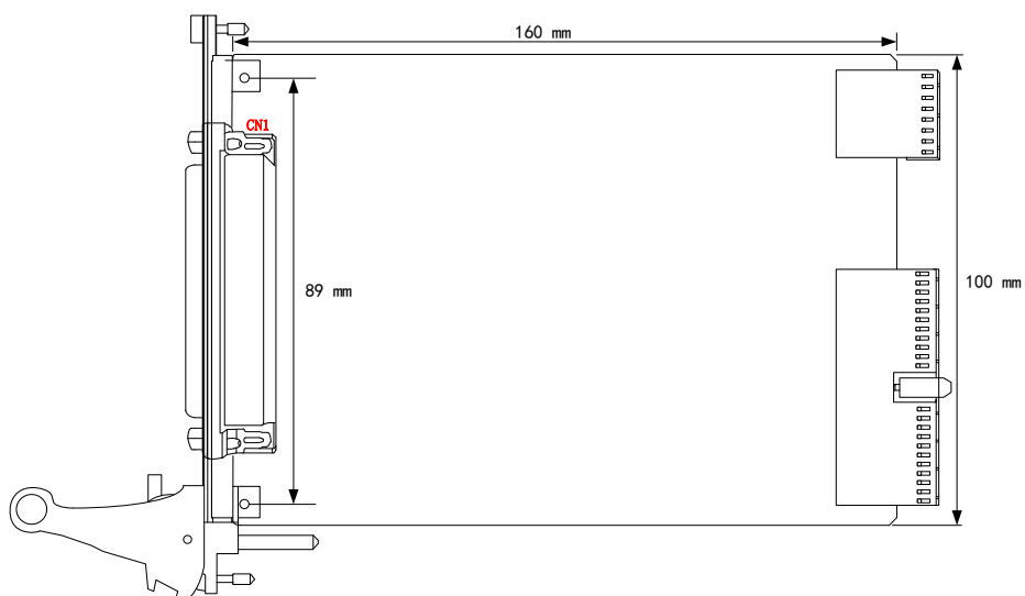
图 3-1-2 PXI2611 尺寸图
