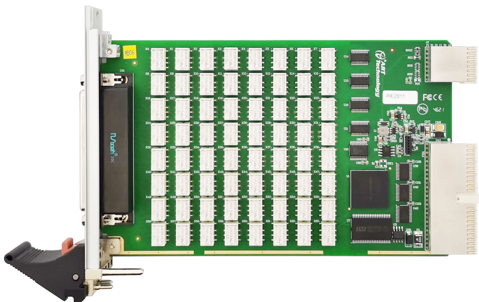
图 3-1-1 PXI2611 外形图
