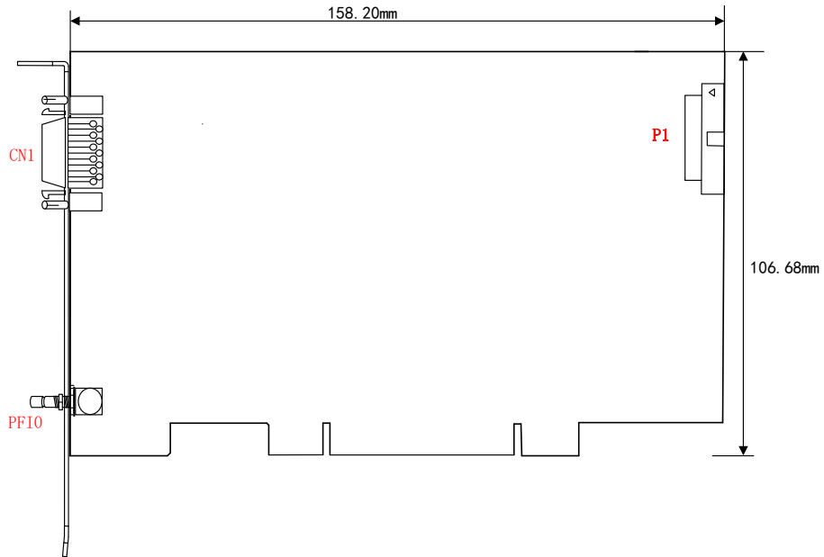
图 3-2-2 PCI8814A 板卡尺寸图
