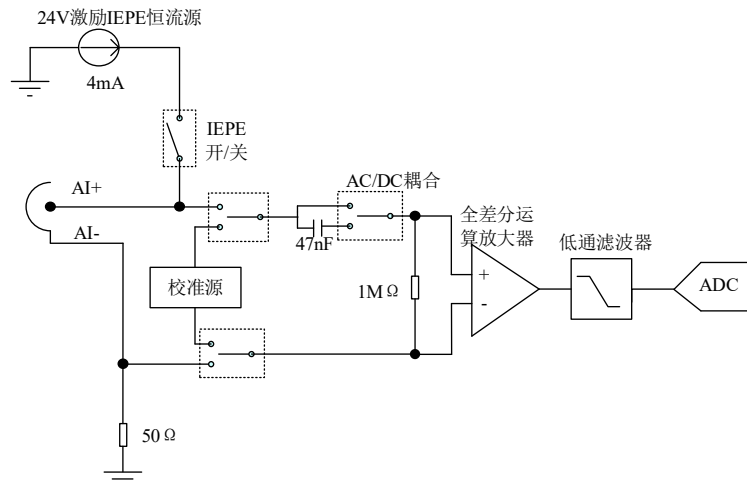
图 4-1-1 模拟输入功能框图
