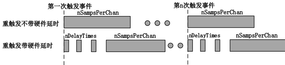
图 4-7-5 AI 重触发
