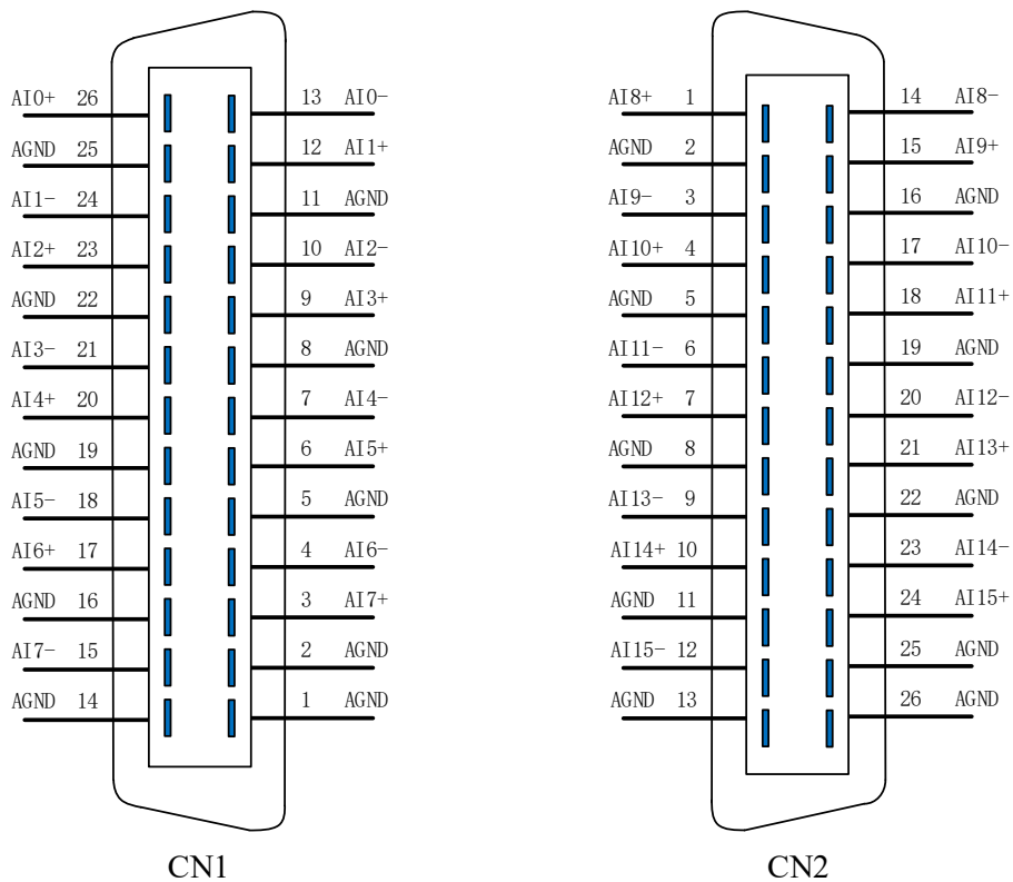
图 3-3-1 PCI8814A / PCI8815 连接器定义图
