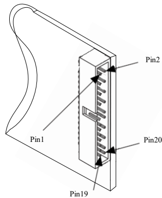
图 3-3-2 RTSI 的 Pinout 图
