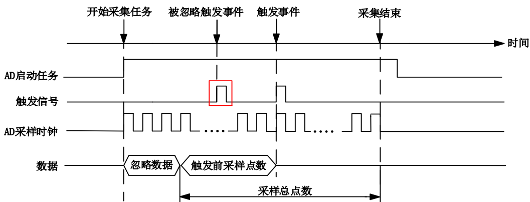
图 4-7-8 参考触发
