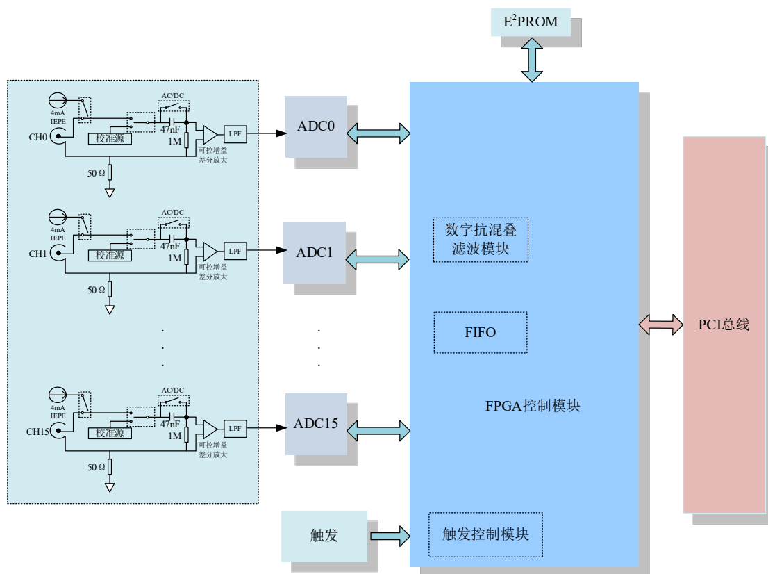
图 2-2-1 PCI8814A / PCI8815 系统框图
