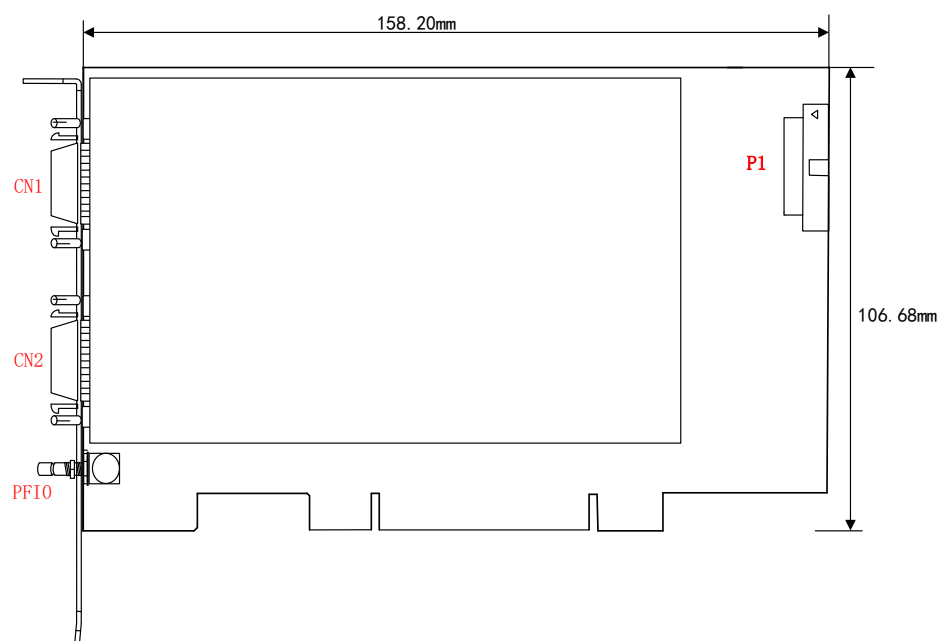
图 3-2-1 PCI8815 板卡尺寸图
