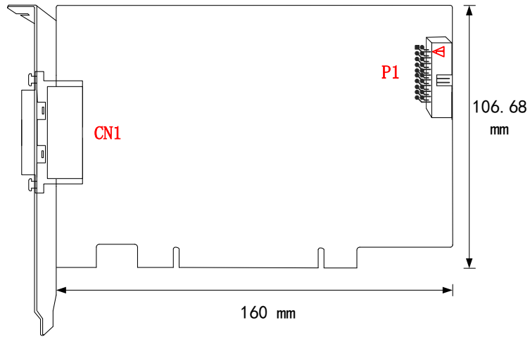
图 3-2-1 PCI9009E 板卡尺寸图
