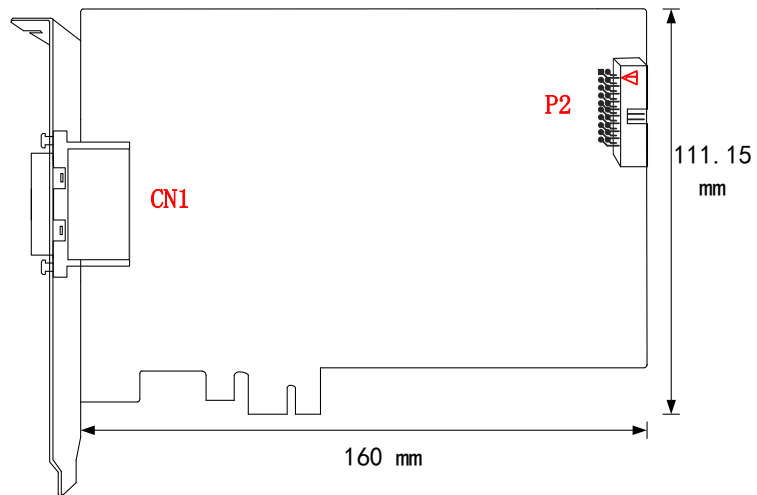
图 3-2-2 PCIe9009E 板卡尺寸图
