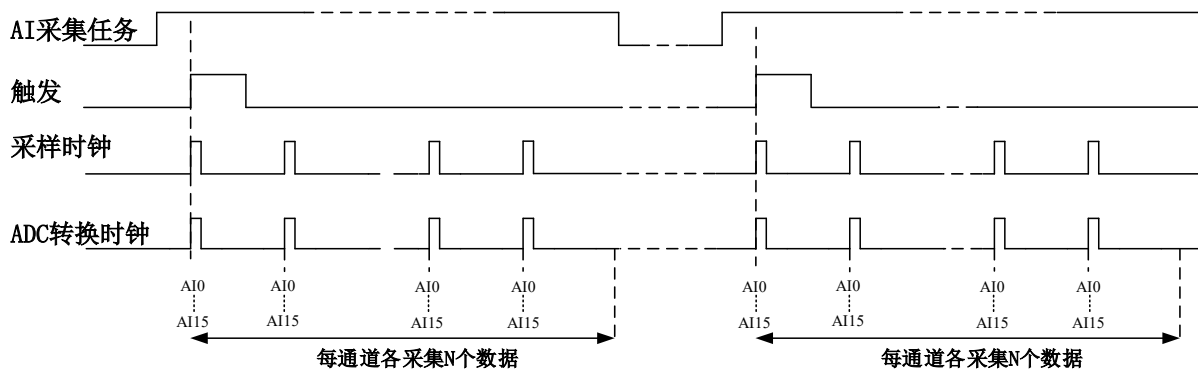
图 4-7-2 有限点采样
