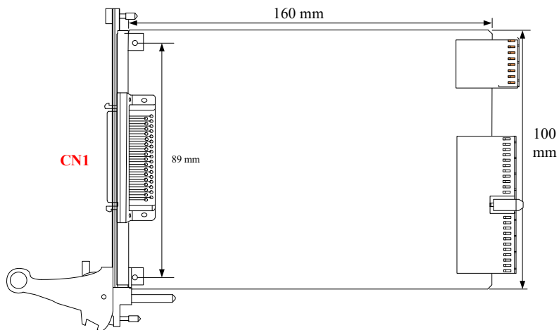
图 3-2-3 PXI9009E 板卡尺寸图
