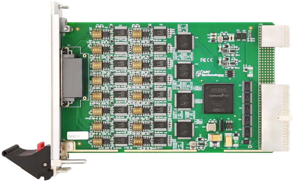
图 3-1-1 PXI6210 外形图
