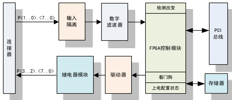
图 2-2-1 PCI2367 系统框图
