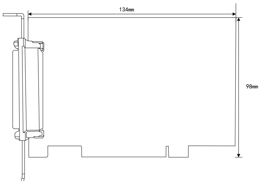
图 3-2-1 PCI2367 尺寸图
