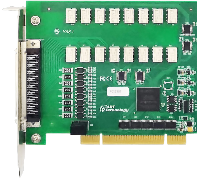
图 3-1-1 PCI2367 外观图
