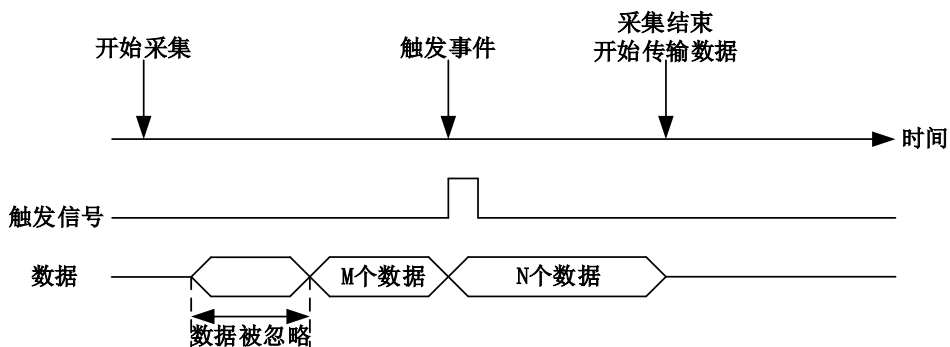
图 4-9-2-2 中间触发
