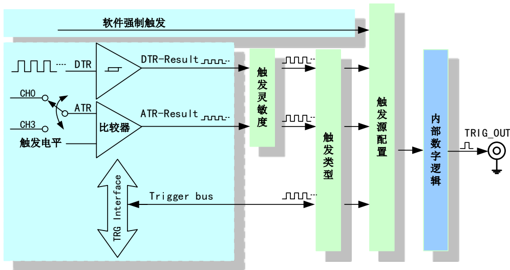
图 4-8-1 AD 触发功能框图
