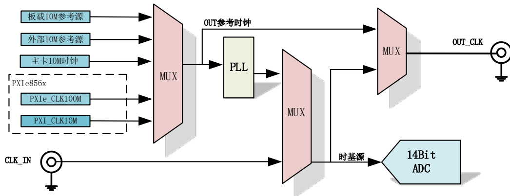
图 4-7-1 856x 时基源框图
