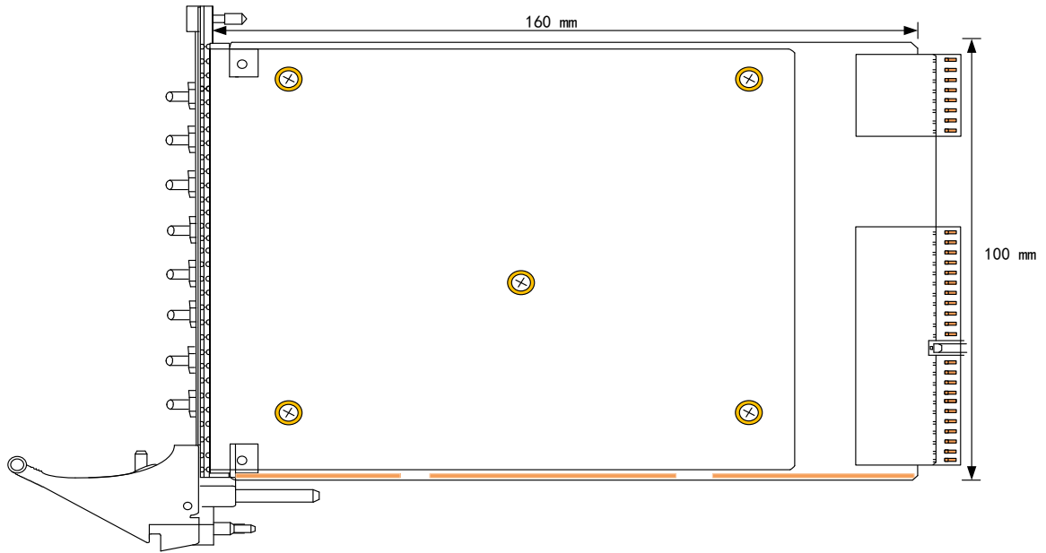
图 3-2-1 PXIe856x 板卡尺寸图
