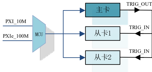
图 4-10-3 采用 PXIe 机箱背板时钟信号作为时钟参考源
