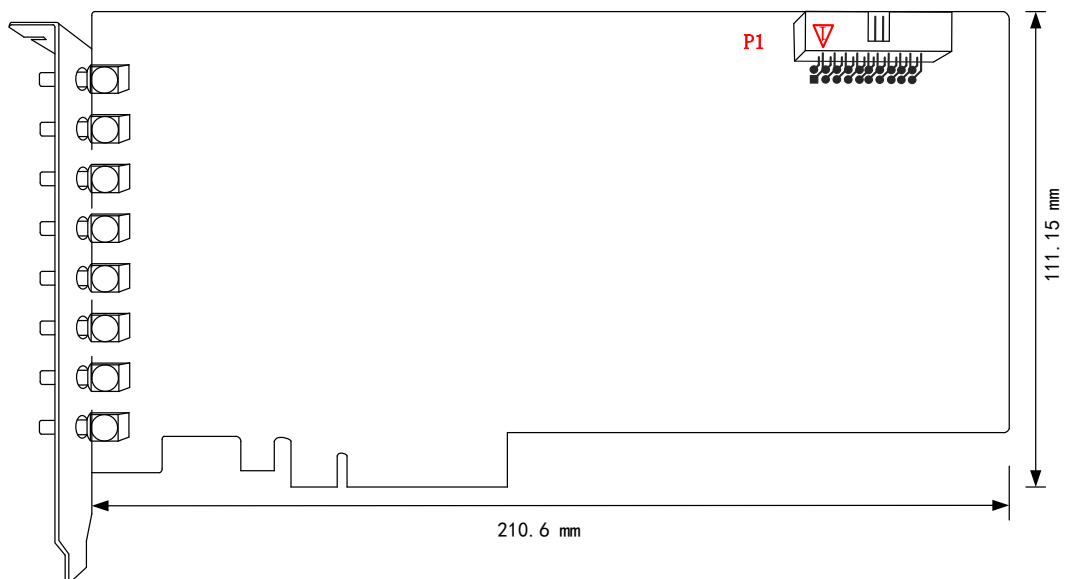
图 3-2-1 PCIe856x 板卡尺寸图
