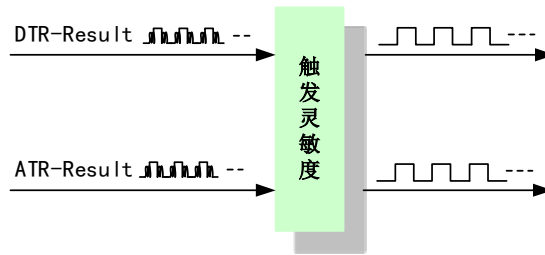
图 4-8-2 触发灵敏度
