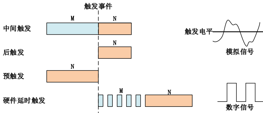
图 4-9-2-1 AD 触发模式
