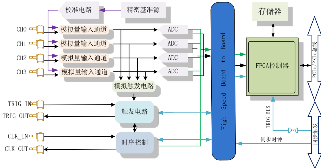
图 3-1-1 856x 系统框图
