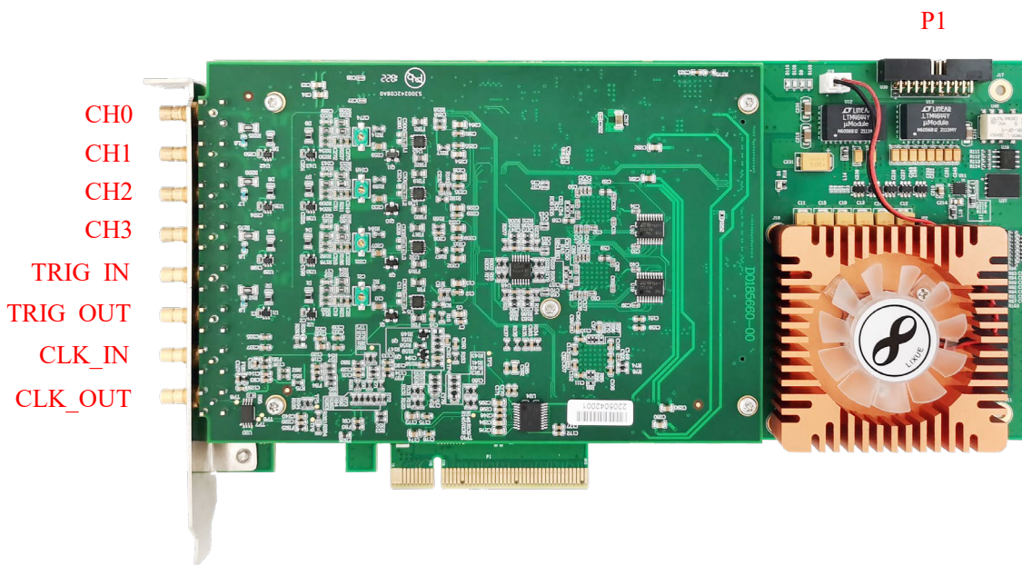
图 3-3-1 PXIe856x 产品外观图
