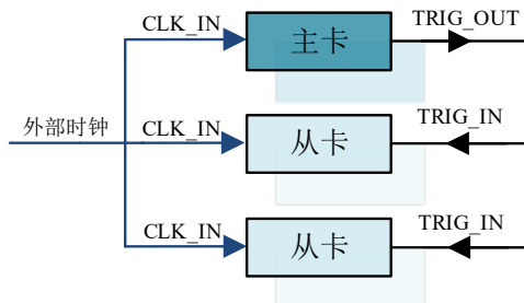
图 4-10-2 采用共同外时钟
