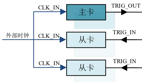
图 4-10-4 共同的外时钟
