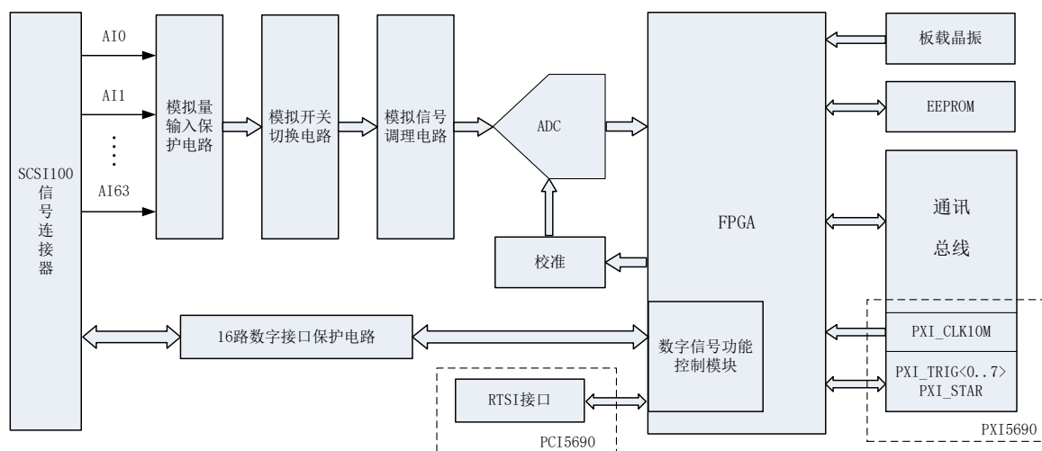
图2-2-1 5690系统框图
