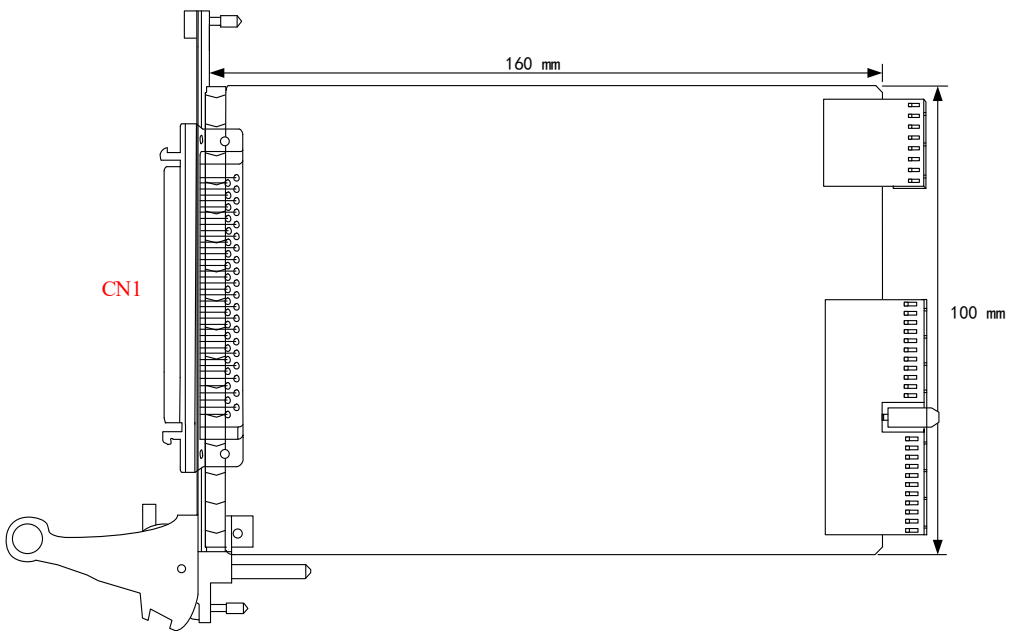
图 3-2-2 PXI5690 板卡尺寸图
