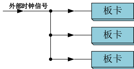
图4-10-6 外时钟同步采集的连接方式
