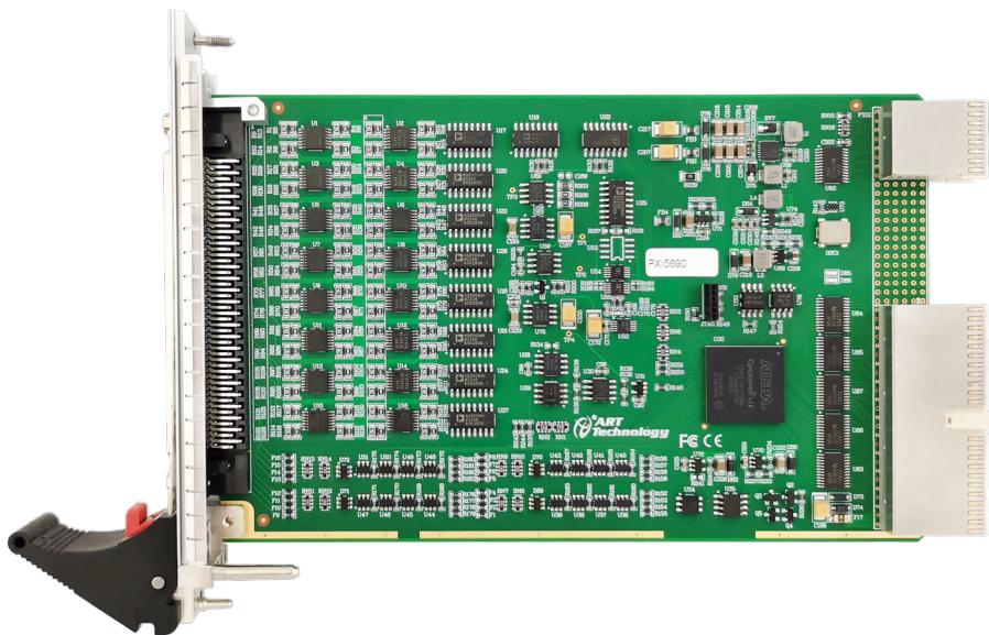
图 3-1-2 PXI5690 正面图
