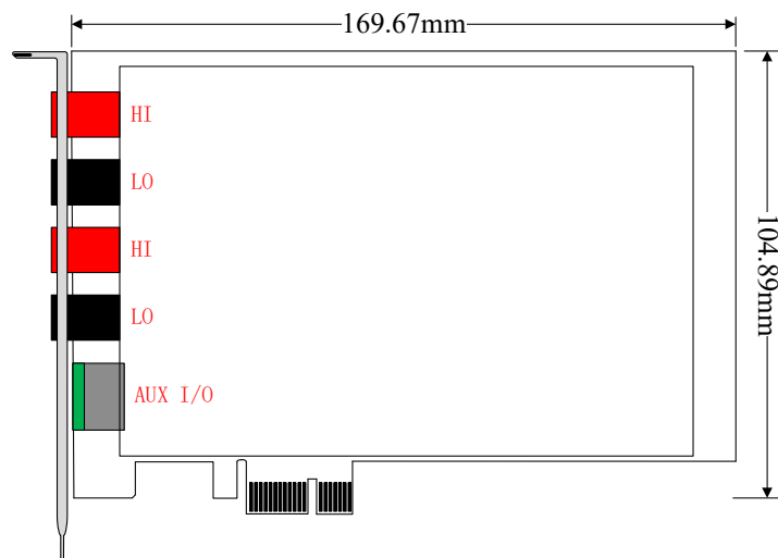
图 3-2-4 PCIe7065 板卡尺寸图
