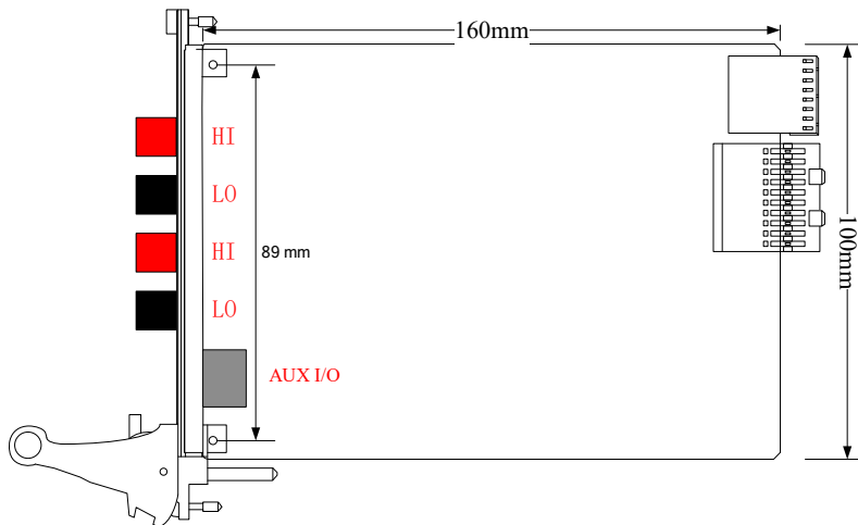
图 3-2-1 PXI7065 板卡尺寸图
