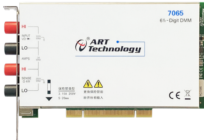
图 3-1-2 PCI7065 板卡外形图
