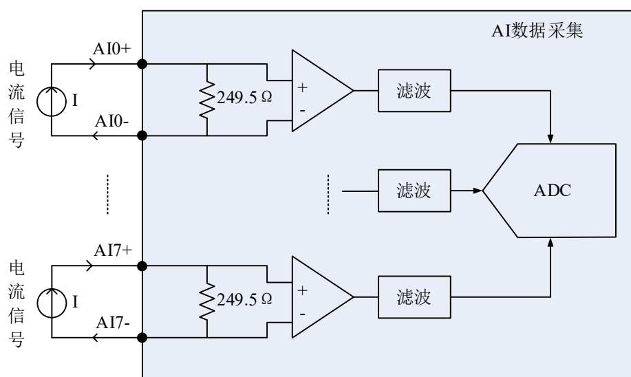
图 4-5-1 电流信号连接方式
