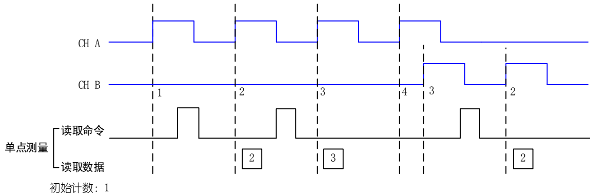
图 5-7-4 双脉冲编码
