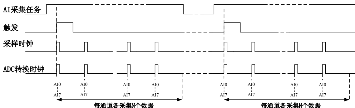
图 4-7-2 有限点采样
