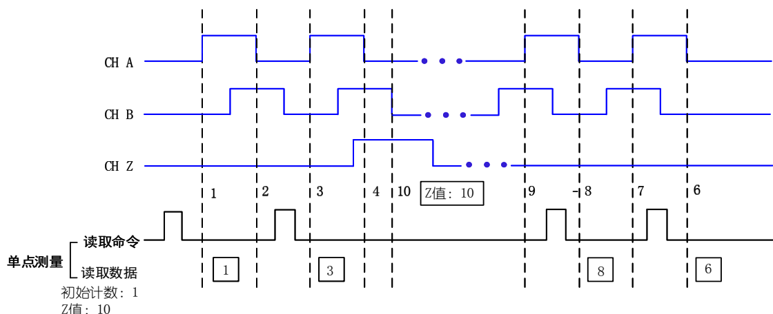
图 5-7-6 Z 索引
