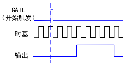
图 5-8-2 具有开始触发的单脉冲生成
