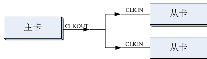
图 4-9-1 主从卡级联同步采集的连接方式
