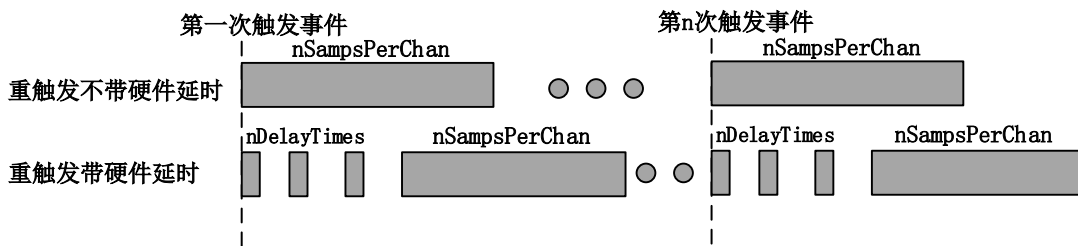
图 7-2-6 AI 重触发
