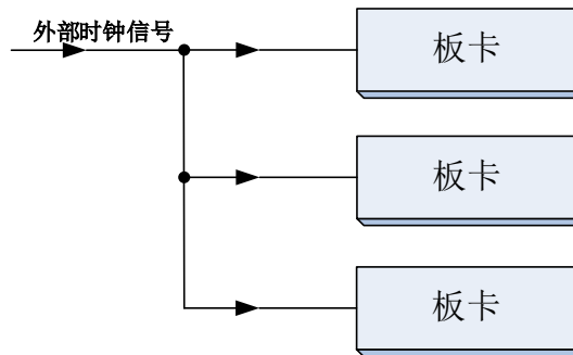
图4-9-3 外时钟同步采集的连接方式
