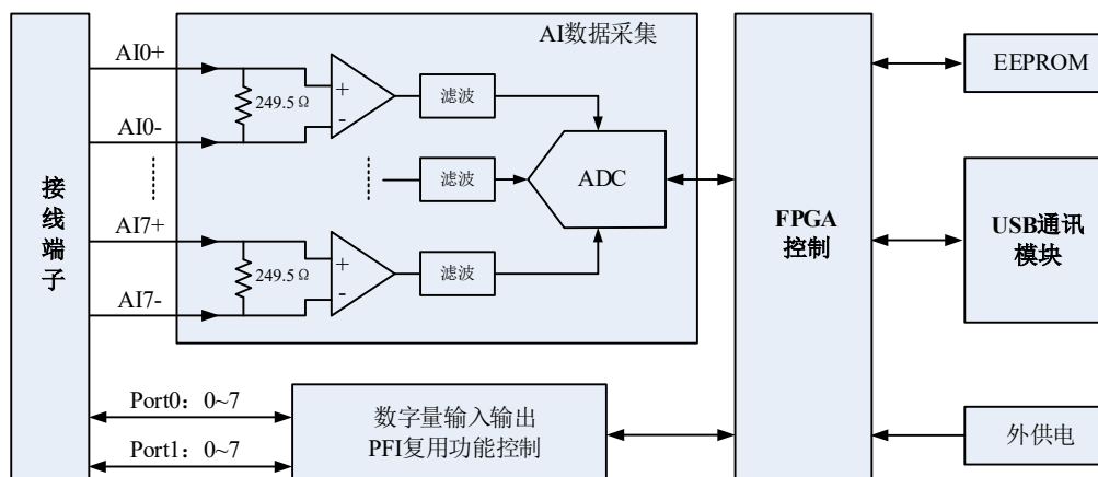
图2-2-1 USB3145A系统框图
