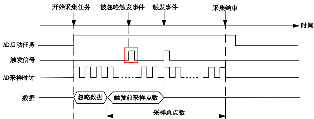
图 7-2-9 参考触发
