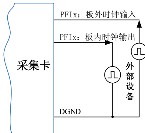
图 4-6-1 时钟输入输出的连接
