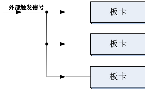
图 4-9-2 外触发同步采集的连接方式
