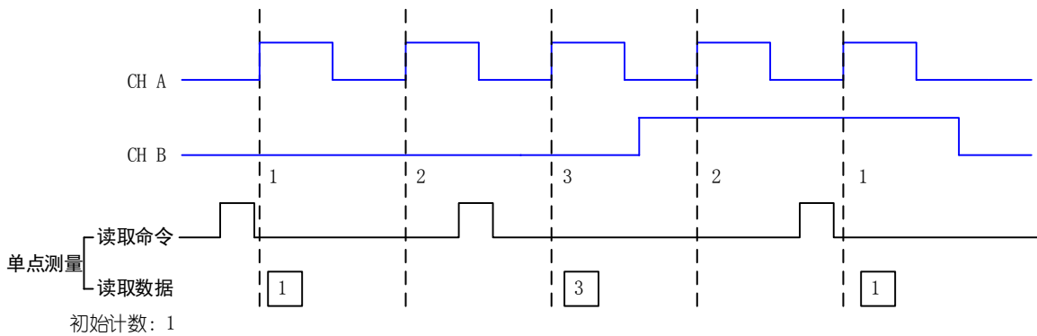
图 5-7-5 单脉冲编码
