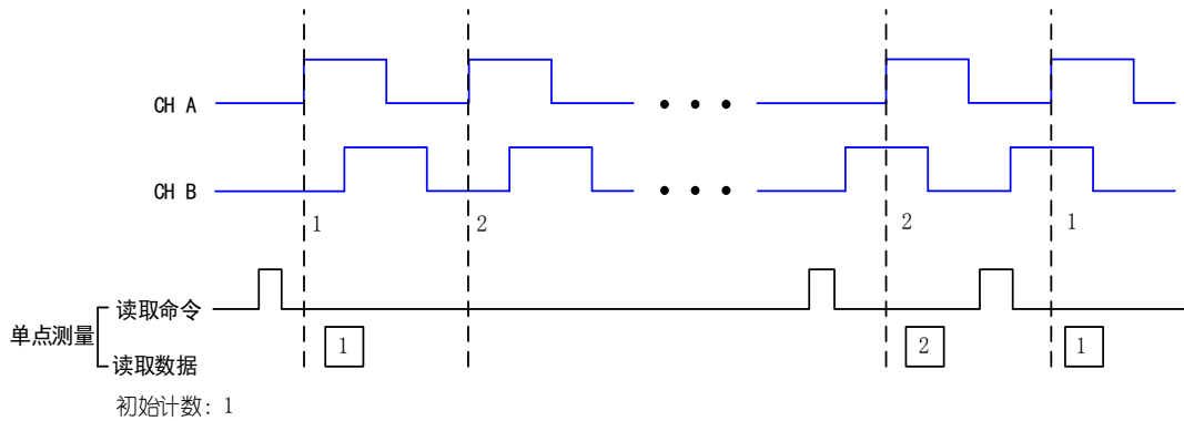
图 5-7-1 X1 编码
