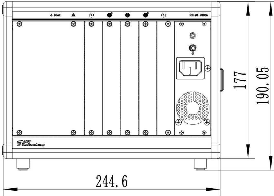
图 1 产品正视图
