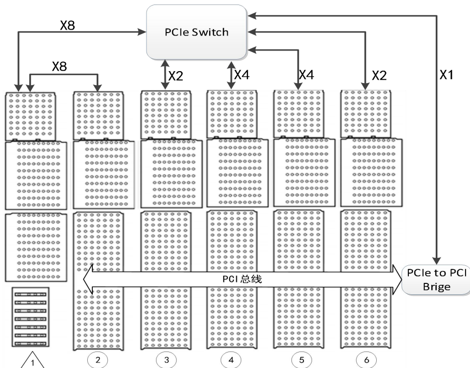
图 4 总线拓扑图
