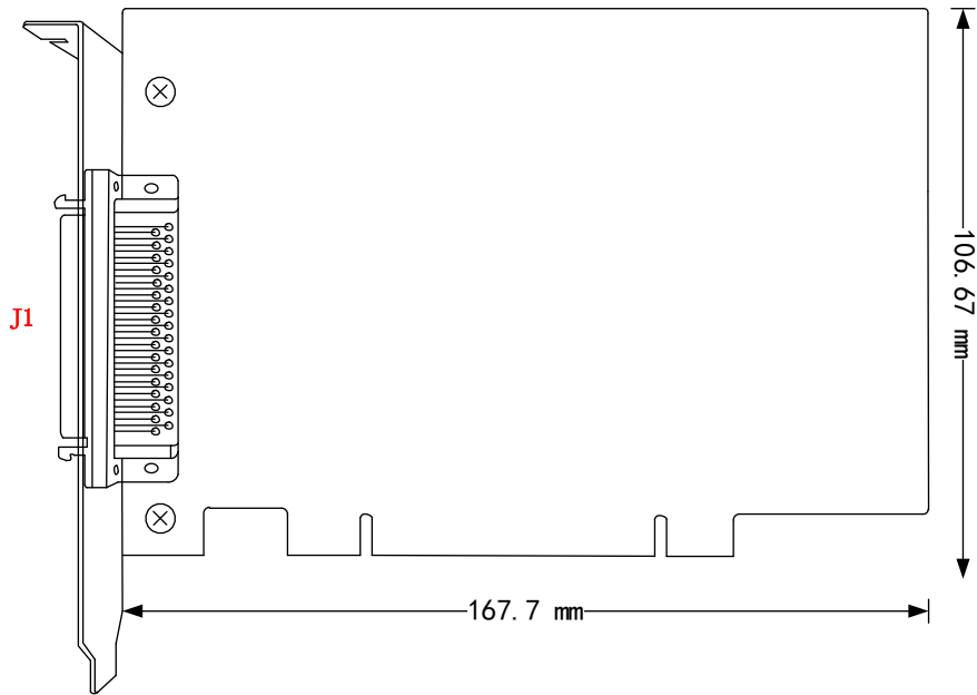
图 3-2-1 PCI565x 板卡尺寸图
