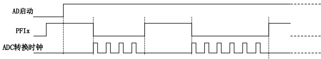
图 8-2-8 暂停触发—高电平暂停
