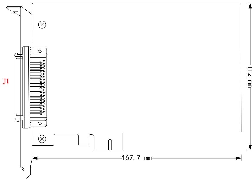
图 3-2-2 PCIe565x 板卡尺寸图
