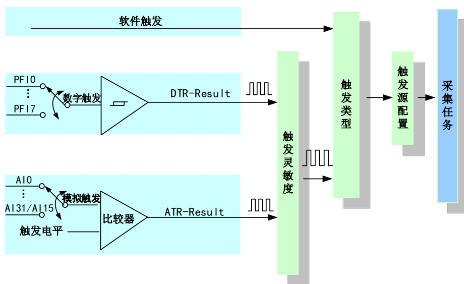
图 8-1-1 触发源选择
