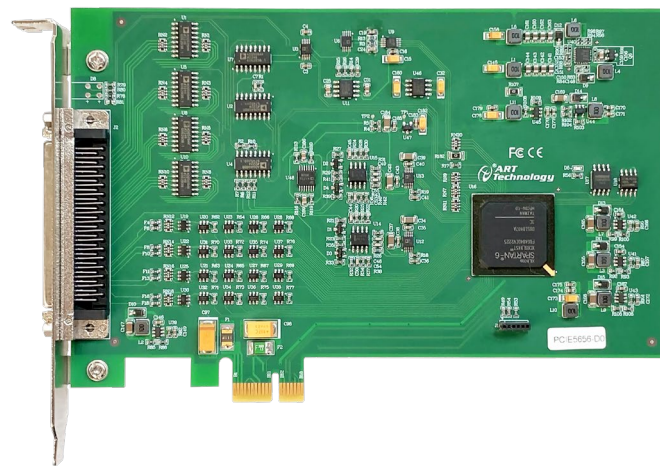
图 3-1-2 PCIe565x 正面图
