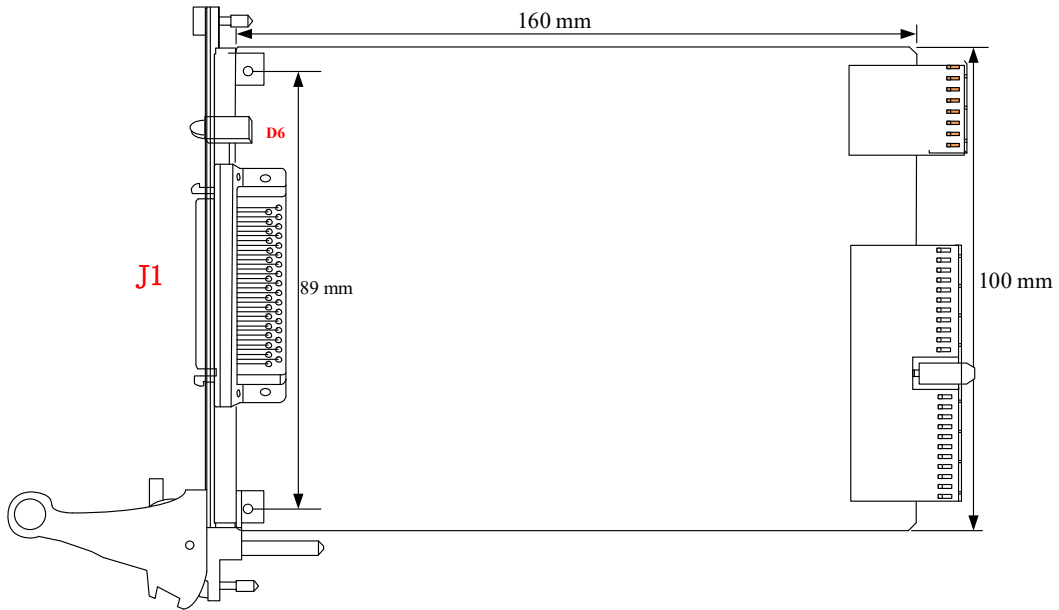
图 3-2-3 PXI565x 板卡尺寸图
