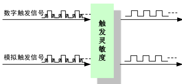
图 8-1-2 触发灵敏度
