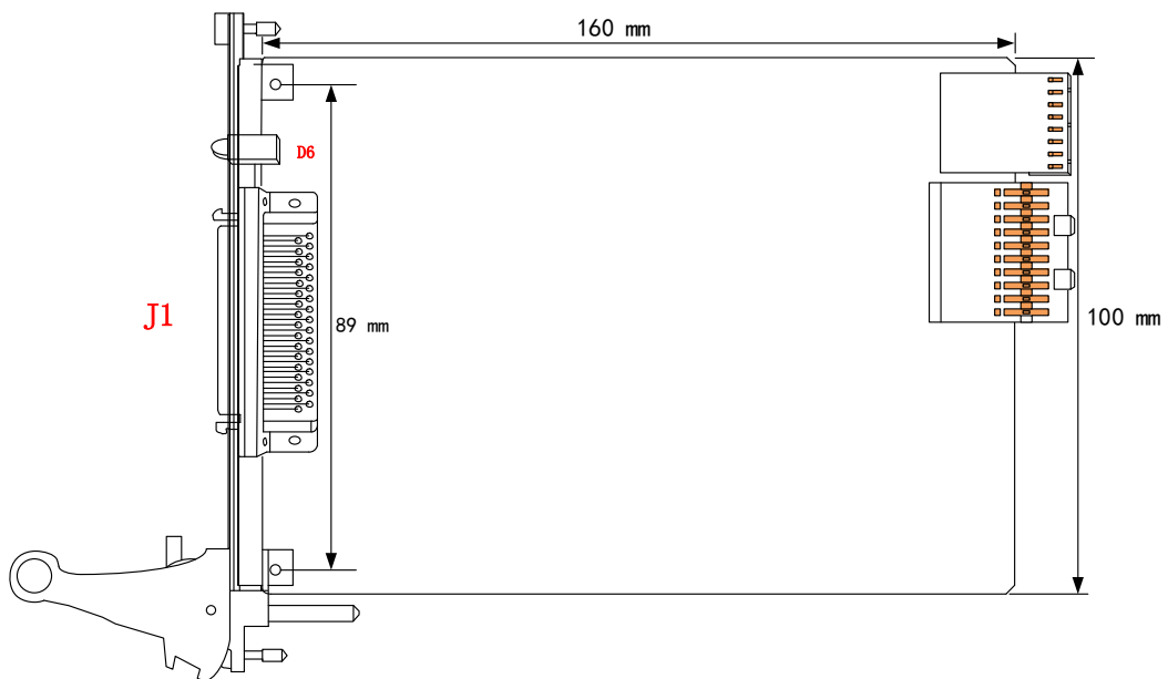
图 3-2-4 PXIe565x 板卡尺寸图
