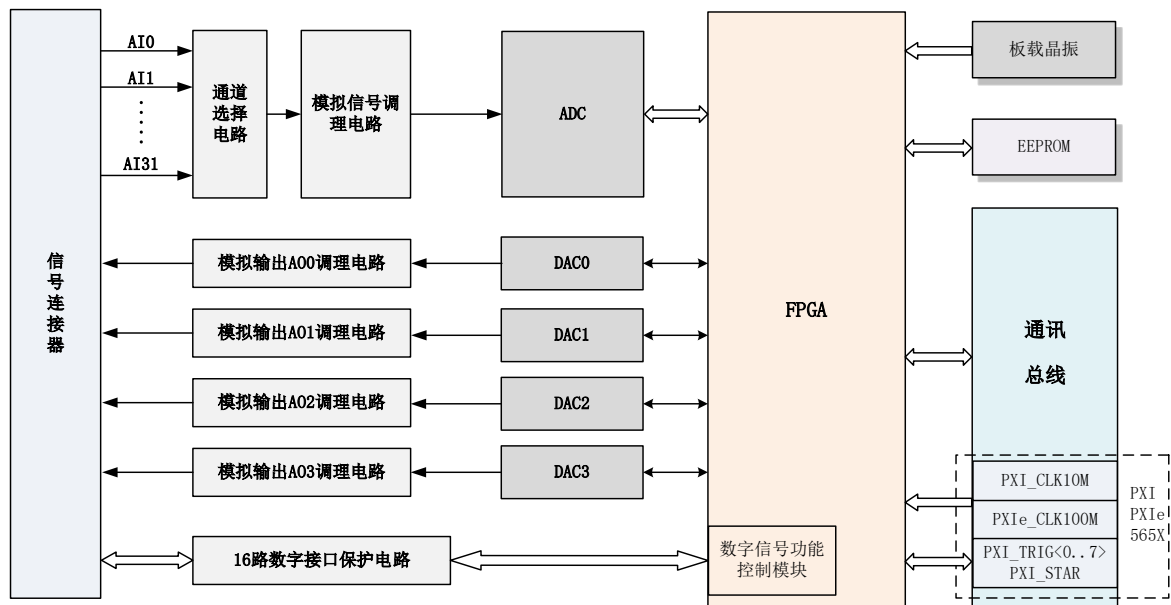
图2-2-1 565X系统框图
