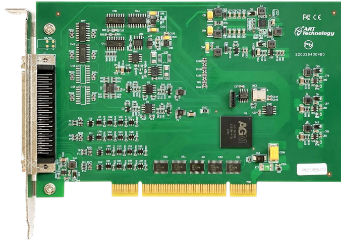
图 3-1-1 PCI565x 正面图
