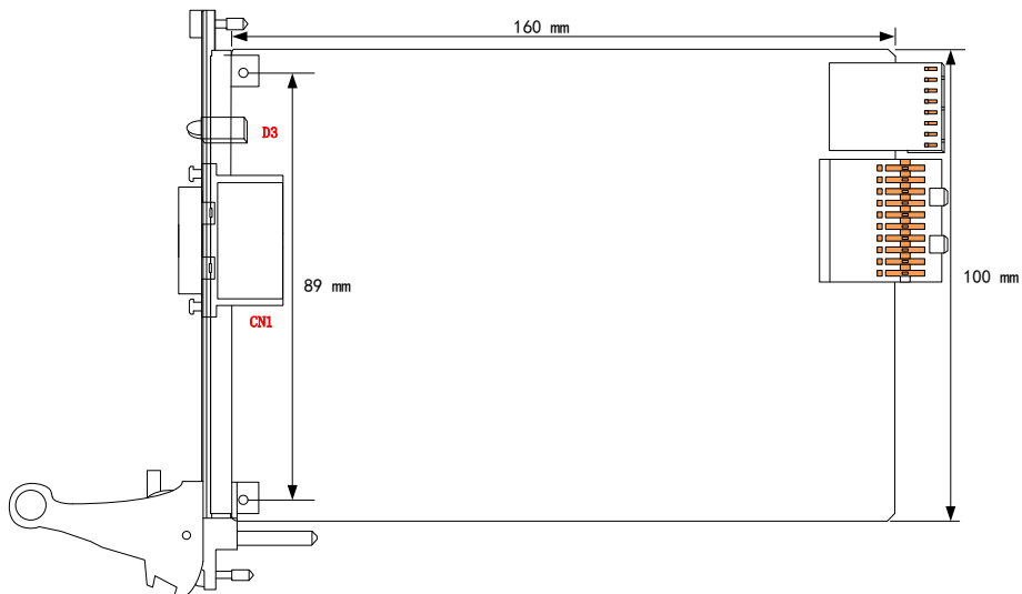
图 3-2-2 PXIe932X 板卡尺寸图
