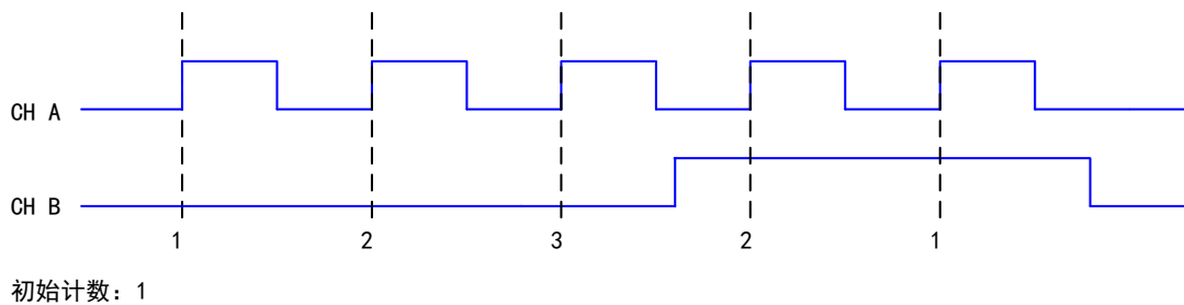
图 6-7-5 单脉冲编码
