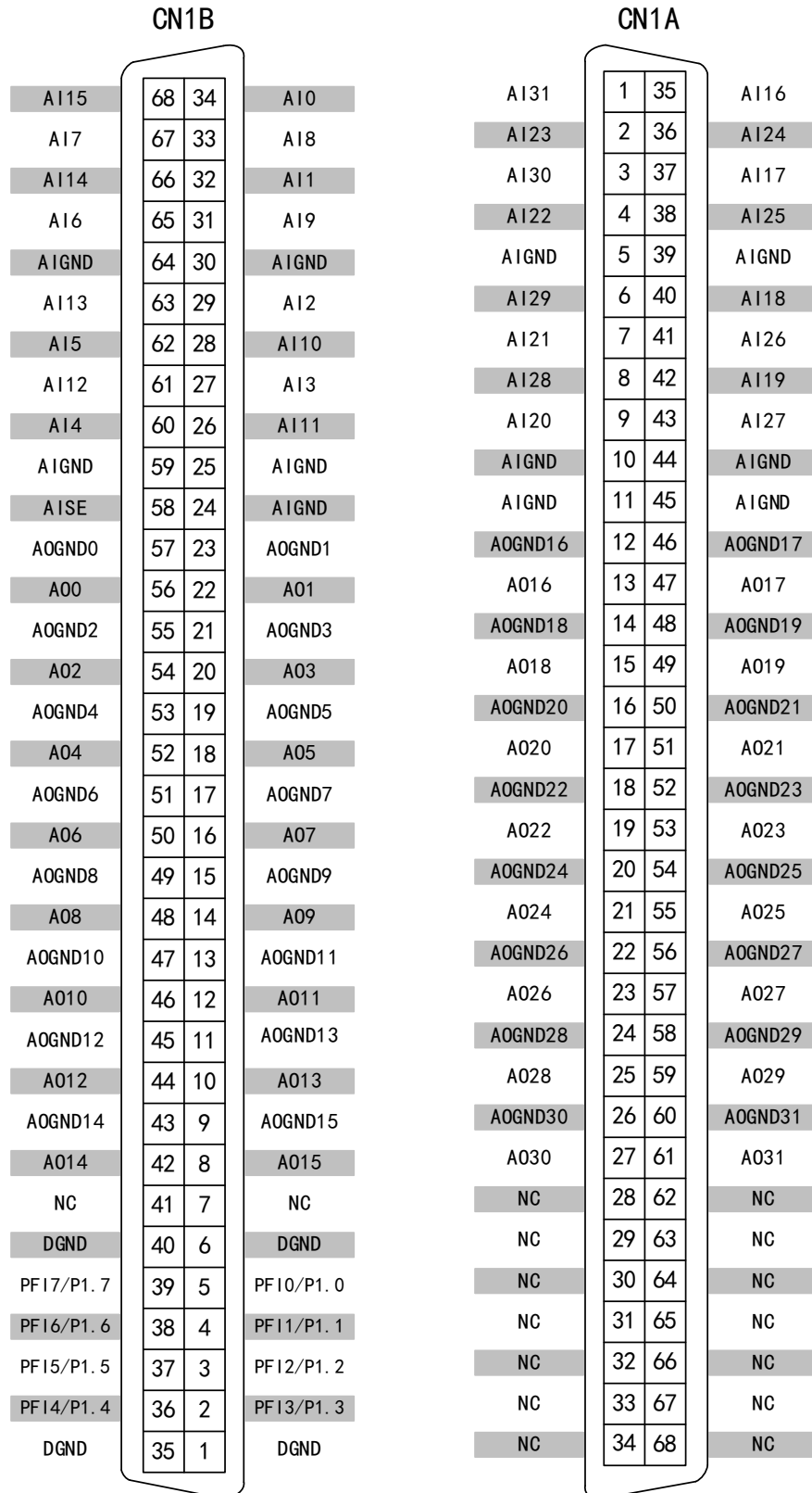
图 3-3-3 9320 连接器引脚定义
