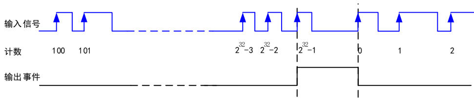
图 5-10-1 脉冲方式输出
