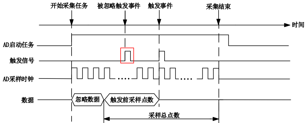
图 4-9-8 参考触发
