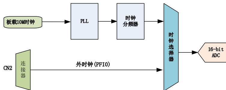
图 4-6-1 AI 时钟结构框图
