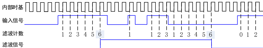
图 5-9-1 数字滤波示例
