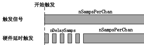
图4-9-3 硬件延时触发方式
