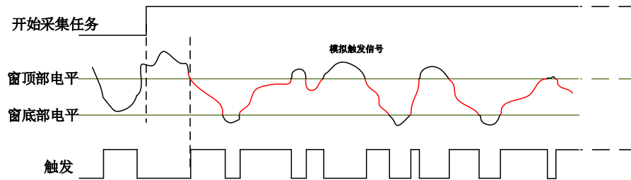
图4-8-7 模拟窗触发--入窗
