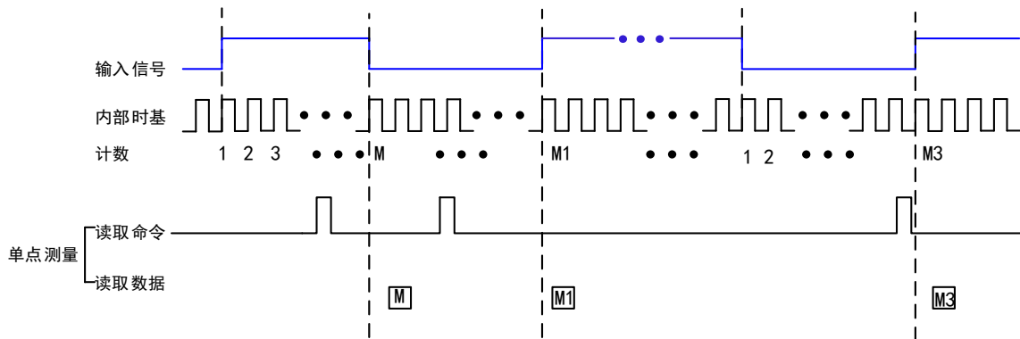
图 5-3-1 半周期示意图
