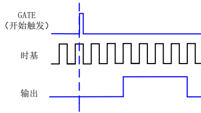
图 5-8-2 具有启动触发的单脉冲生成
