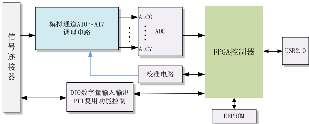
图 2-2-1 USB2889 系统框图
