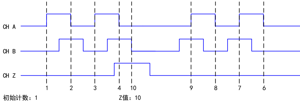
图 5-7-6 Z 索引
