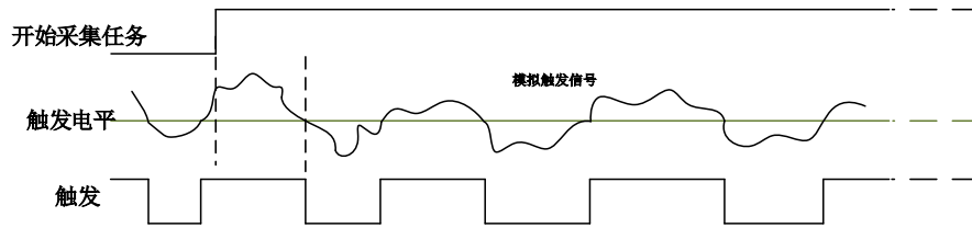
图4-8-6 模拟边沿触发--下降沿触发
