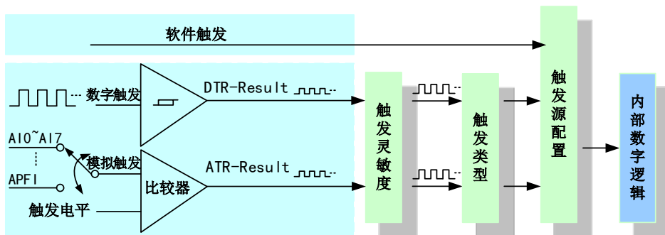
图 4-8-1 AI 触发功能框图
