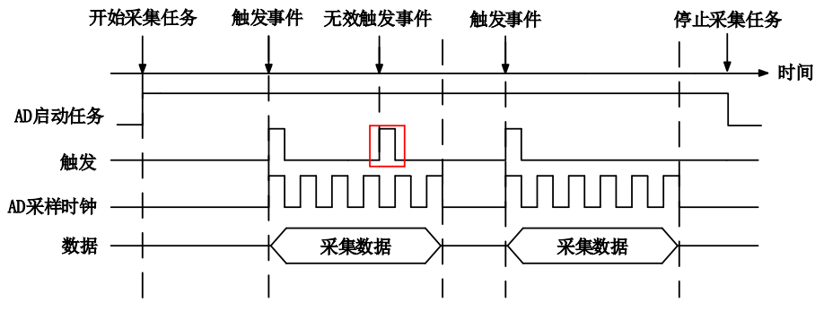
图 4-9-6 重触发
