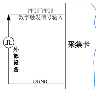
图4-8-8 数字触发连接方法
