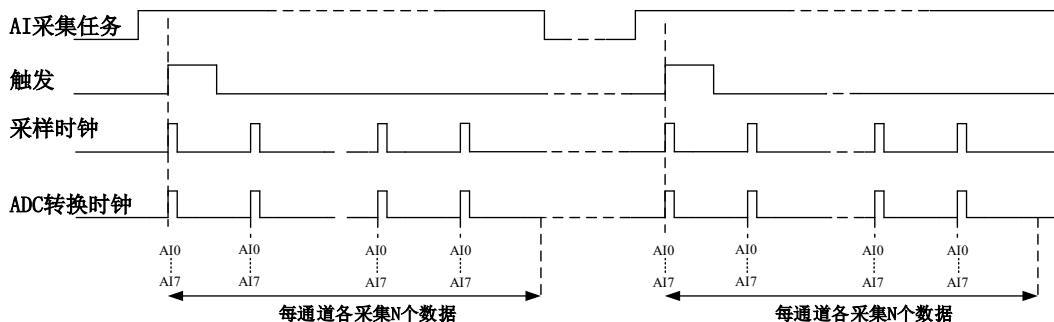
图 4-7-2 有限点采样
