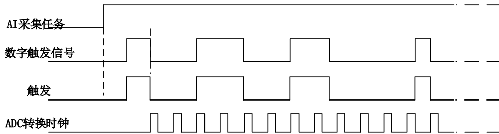
图4-9-2 数字触发--下降沿触发
