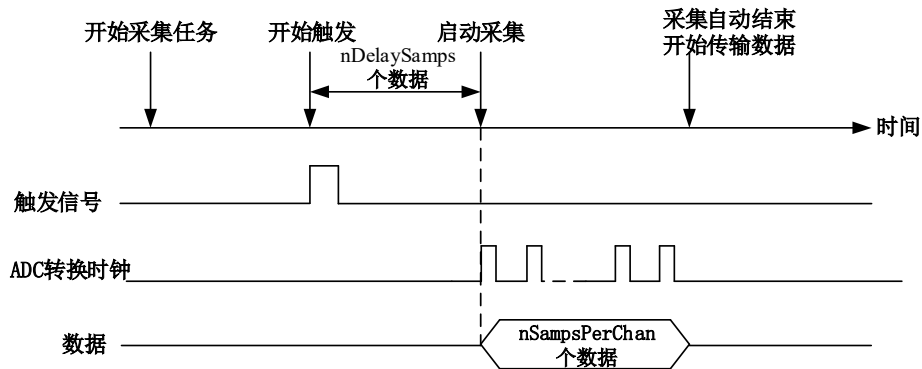
图 4-9-4 硬件延时触发
