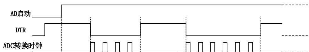
图 4-9-10 暂停触发—高电平暂停
