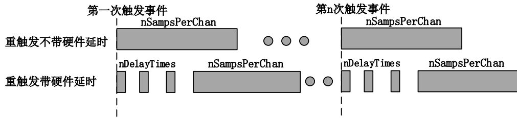
图 4-9-5 AI 重触发
