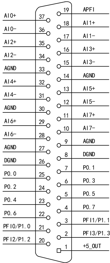
图 3-2-1 USB2889 管脚定义图
