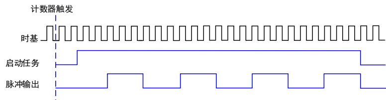
图 5-8-3 有限脉冲序列生成
