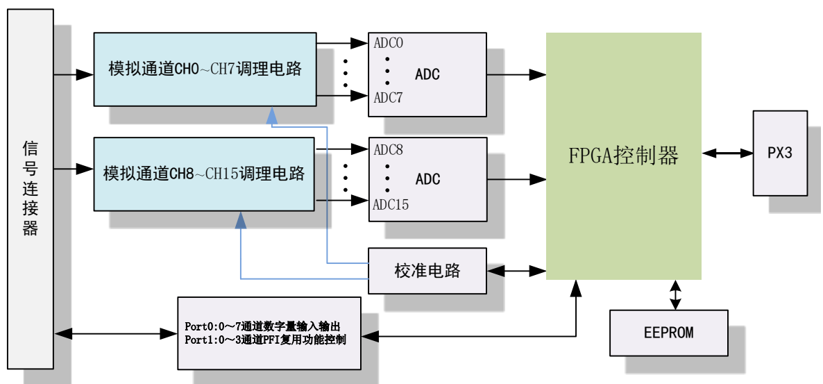
图 2-2-1 USB2880/A/B 系统框图
