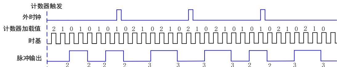
图 5-8-8 有限缓冲外时钟脉冲序列生成
