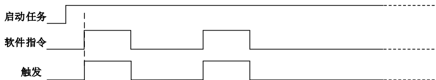
图7-3-2 AI软件强制触发
