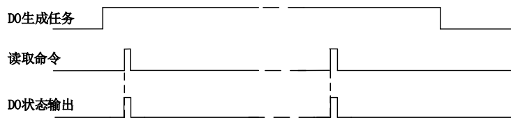
图6-6-1 按需单点生成
