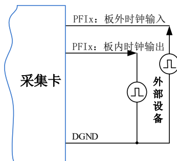
图 6-4-1 时钟输入输出的连接
