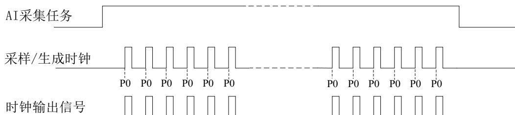
图 6-4-3 外时钟时序图
