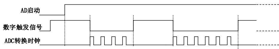
图 7-2-6 暂停触发—高电平暂停
