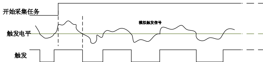
图7-3-5 模拟边沿触发--下降沿触发
