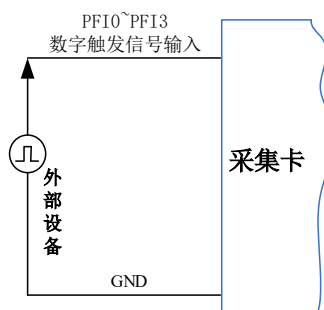
图7-3-8 数字触发连接方法
