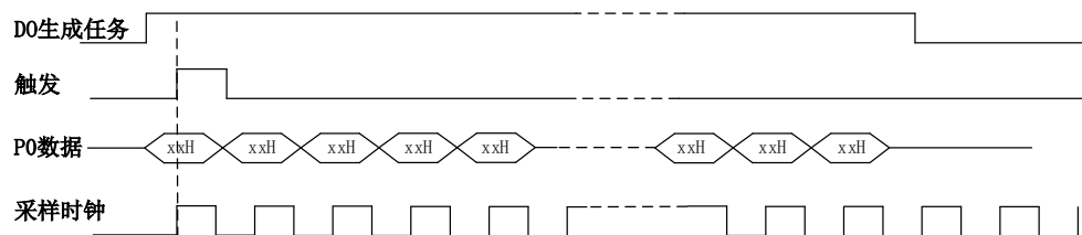
图6-6-3 内、外时钟连续生成
