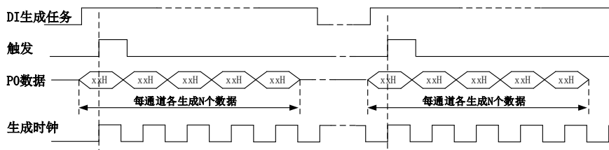
图6-6-2 有限点生成
