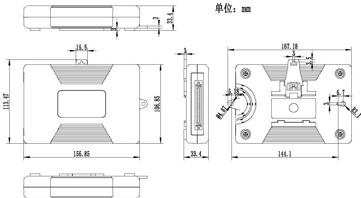
图 3-2-1 USB2880/A/B 外壳尺寸图
