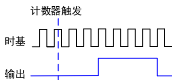
图 5-8-1 单脉冲生成
