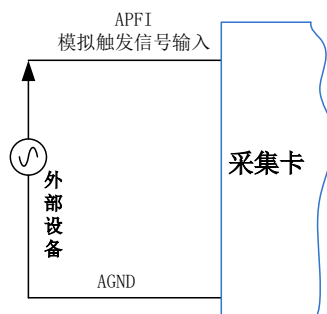
图7-3-3 模拟触发连接方法
