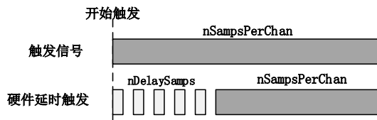
图 7-2-3 AI 硬件延时触发
