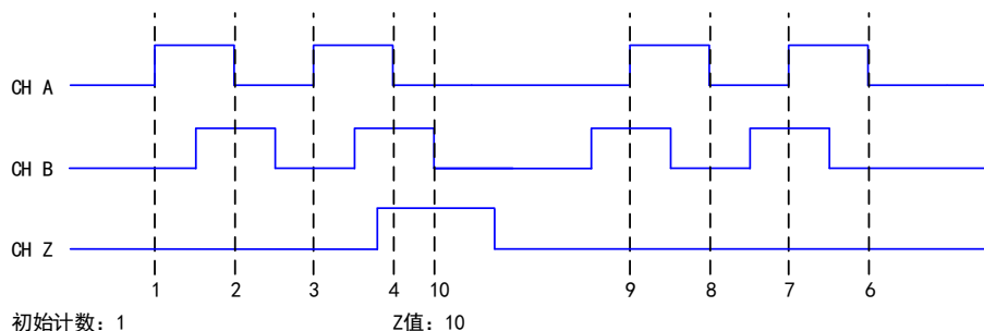
图 5-7-6 Z 索引
