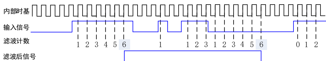
图 5-9-1 数字滤波
