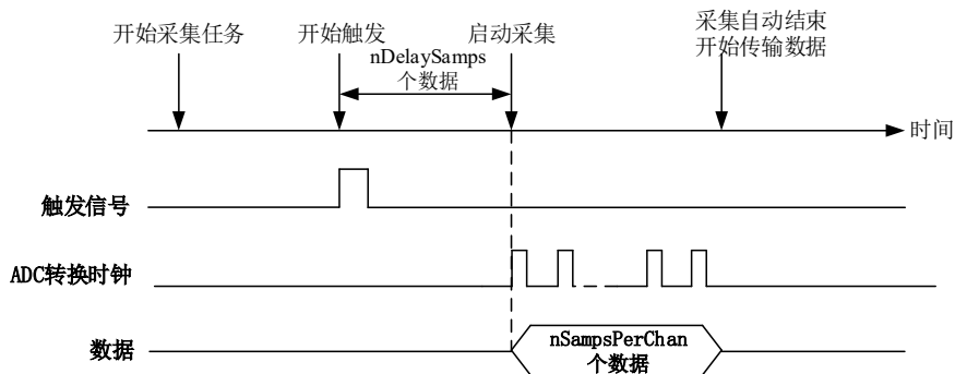
图 7-2-4 硬件延时触发
