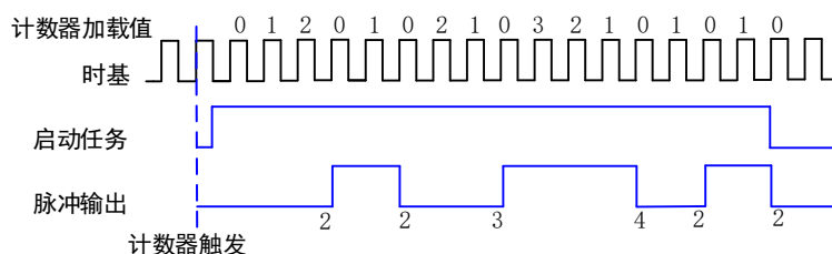
图 5-8-7 有限隐式缓冲脉冲序列生成
