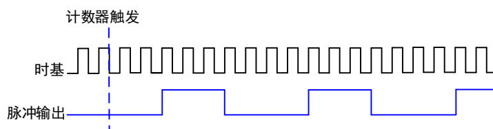
图 5-8-6 连续脉冲序列生成
