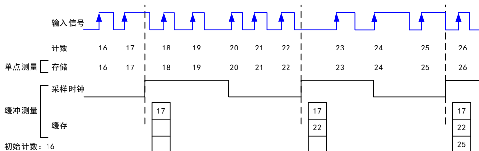
图 5-1-1 边沿加计数上升沿有效示意图
