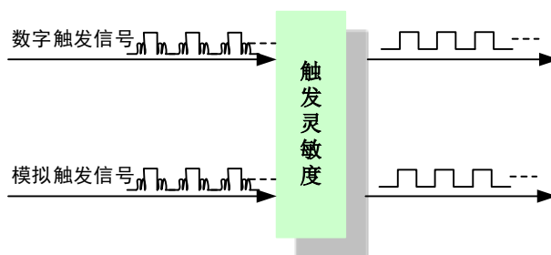
图 7-3-1 触发灵敏度
