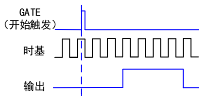
图 5-8-2 具有开始触发的单脉冲生成
