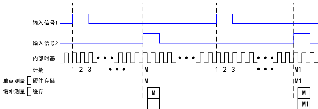
图 5-6-1 两边沿均上升沿有效示意图
