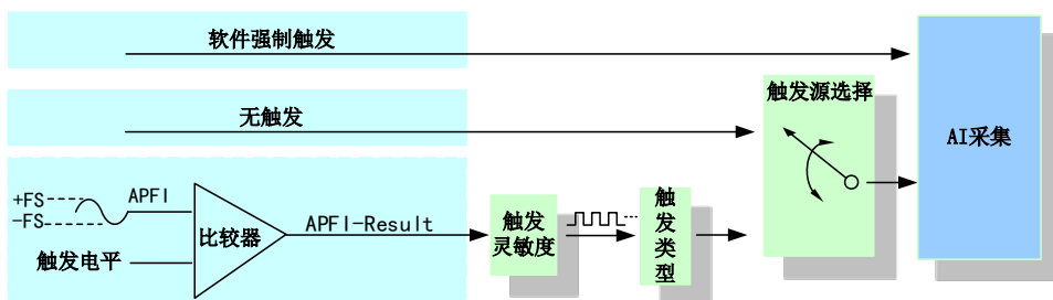
图 7-1-2 模拟触发源选择
