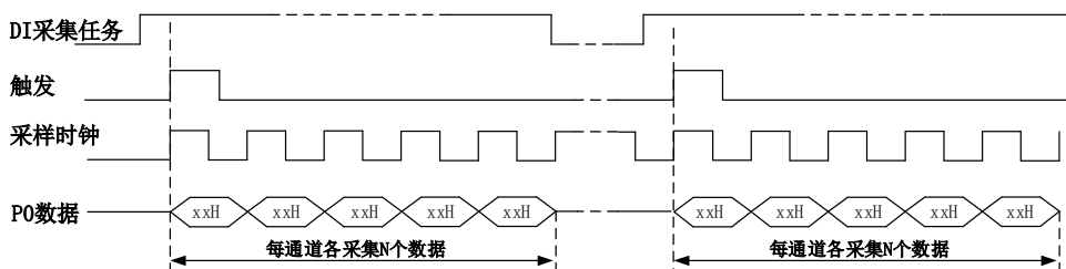
图 6-5-2 有限点采样
