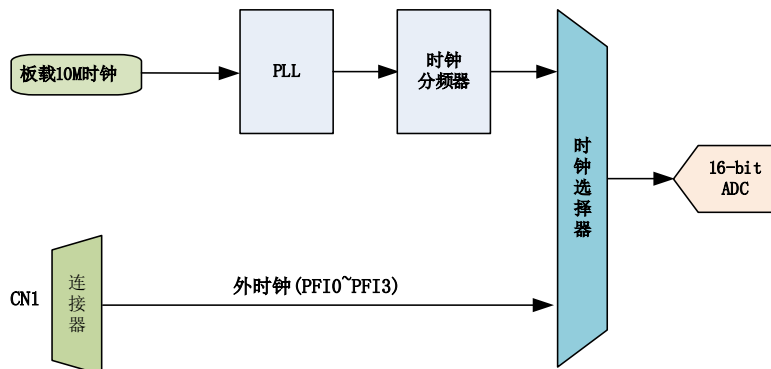
图 4-6-1 AI 时钟结构框图
