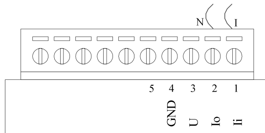
图 9（无电流互感器）
