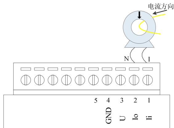
图 10（外置电流互感器）
