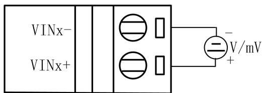
图 6 电压接法
