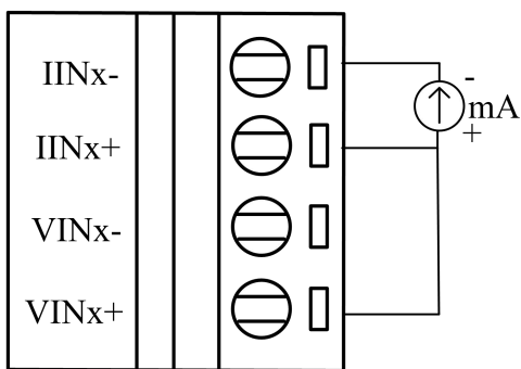
图 5 电流接法
