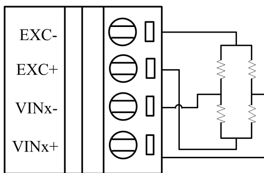
图 8 桥式接法
