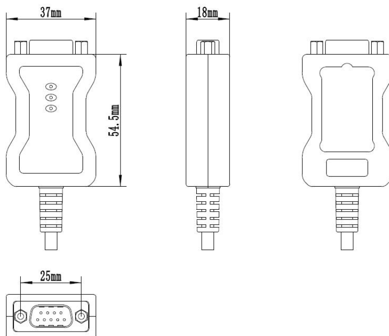
图 2 外壳尺寸图
