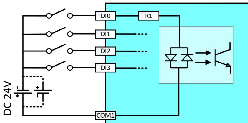
图 2 输入接线
