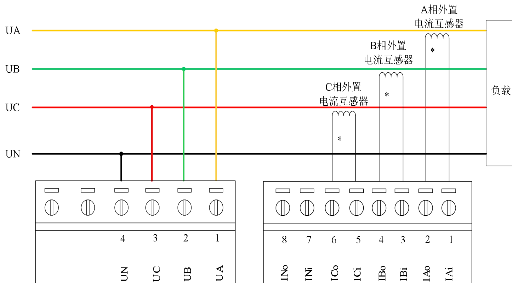
图 9（三相四线电压接线图）
