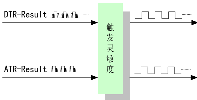
图 4-8-2 触发灵敏度
