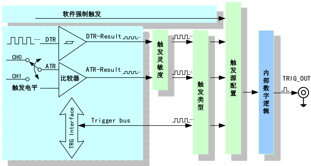
图 4-8-1 AD 触发功能框图
