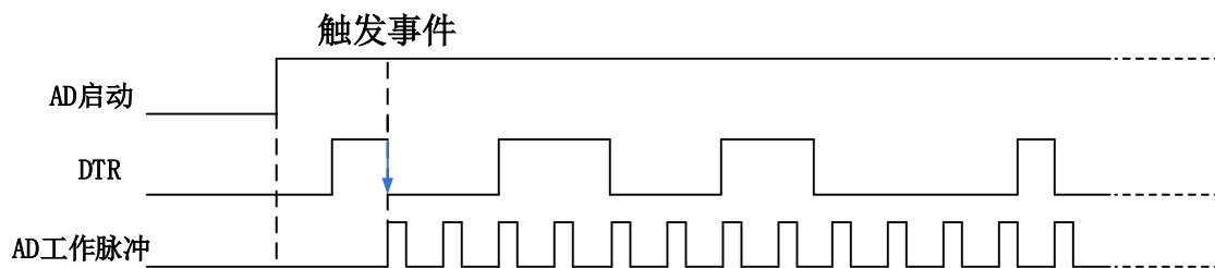
图 4-8-9 DTR 触发--下降沿触发
