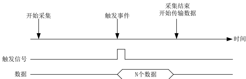
图 4-9-2-2 后触发
