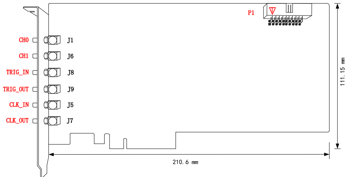
图 3-2-1 PCIe8916A 板卡尺寸图
