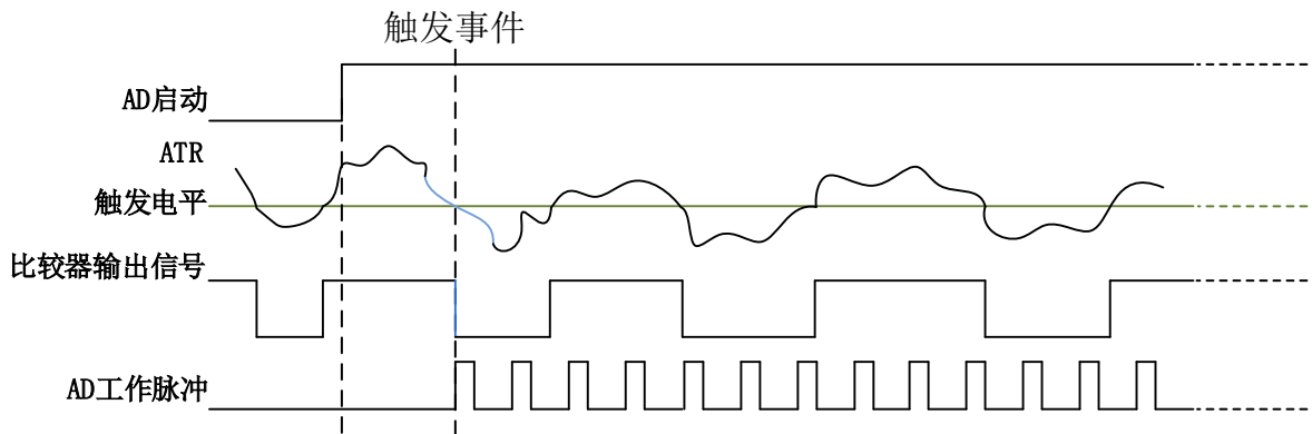
图 4-8-6 ATR 触发--下降沿触发
