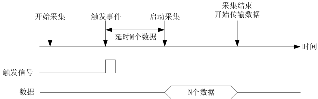
图 4-9-2-3 硬件延时触发
