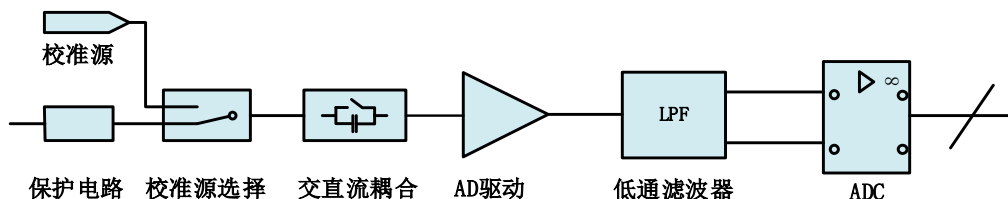
图 4-1-1 AI 功能框图
