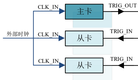
图 4-10-2 共同的外时钟
