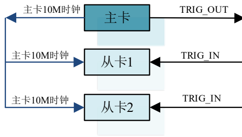
图 4-10-1 主从卡级联
