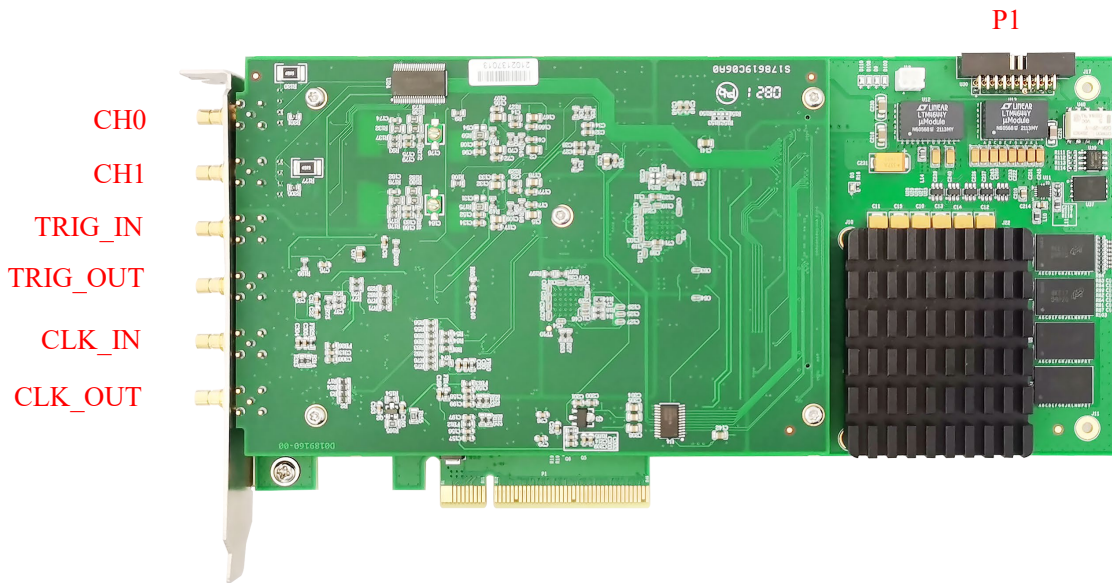
图 3-3-1 PCIe8916A 产品外观图
