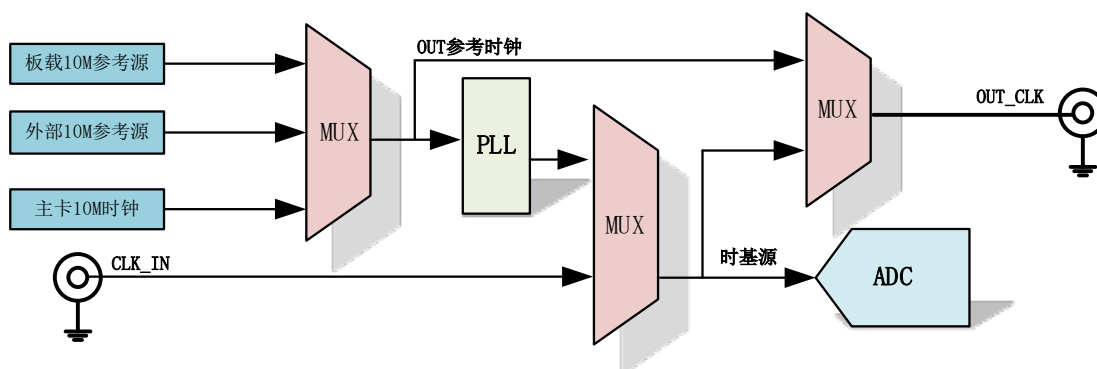
图 4-7-1 时基源框图
