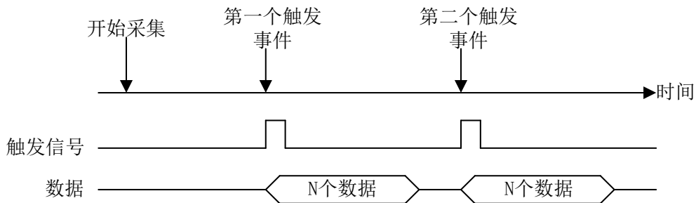
图 4-9-2-4 后触发和延时触发的重复触发
