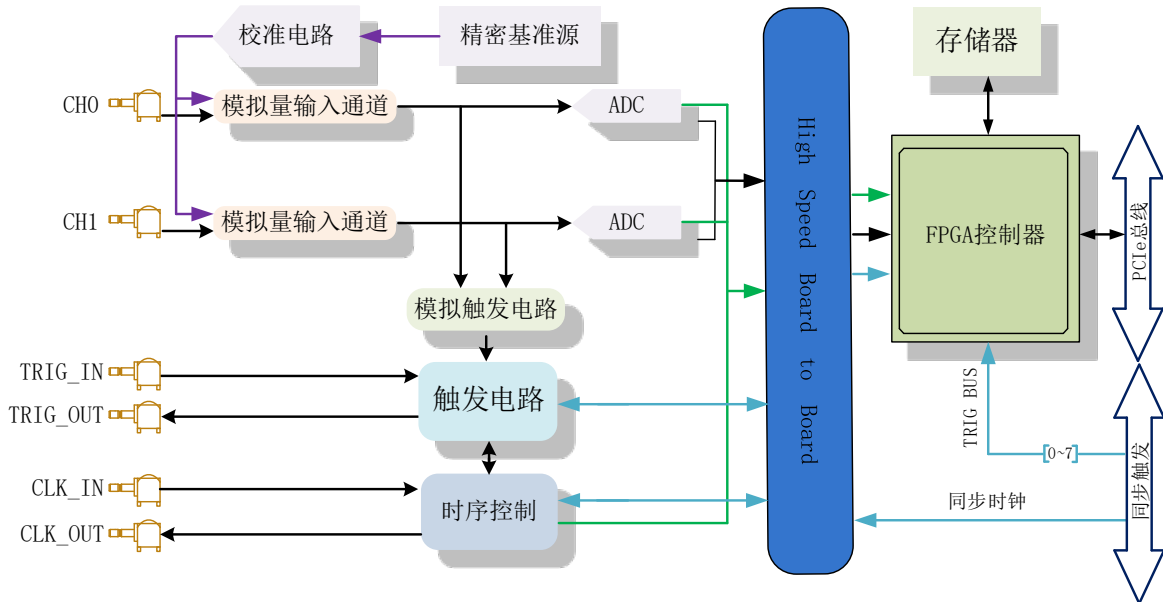
图 3-1-1 PCIe8916A 系统框图
