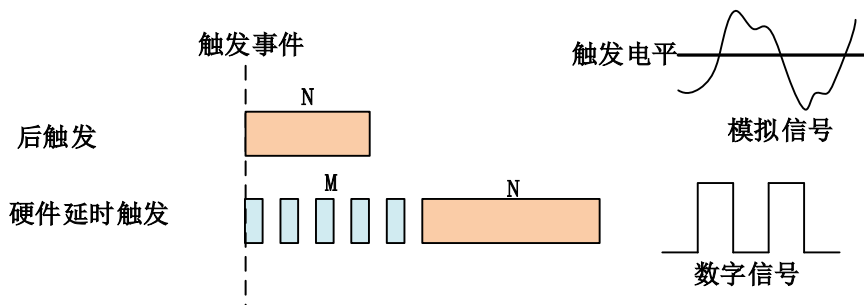
图 4-9-2-1 AI 触发模式
