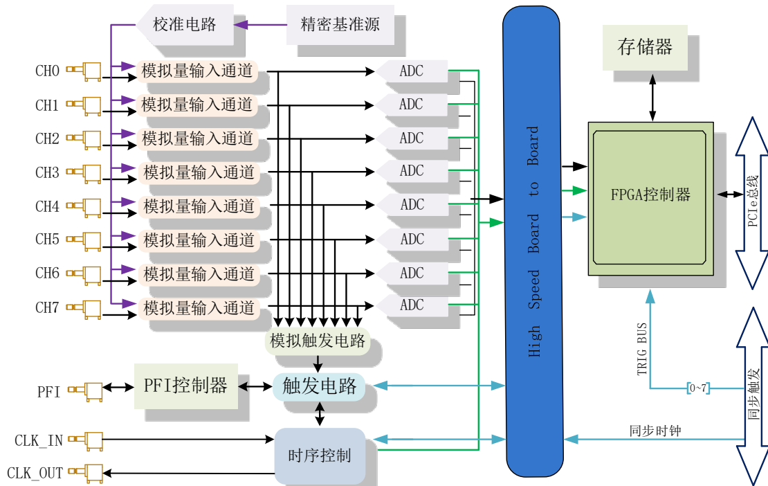
图 3-1-1 PCIe858xA 系统框图
