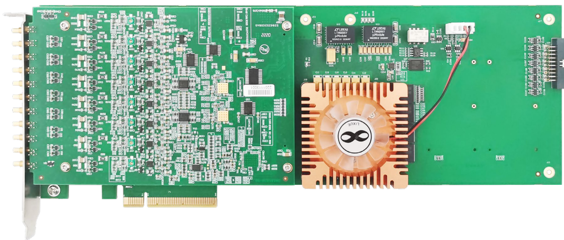
图 3-3-1 PCIe858xA 产品外观图
