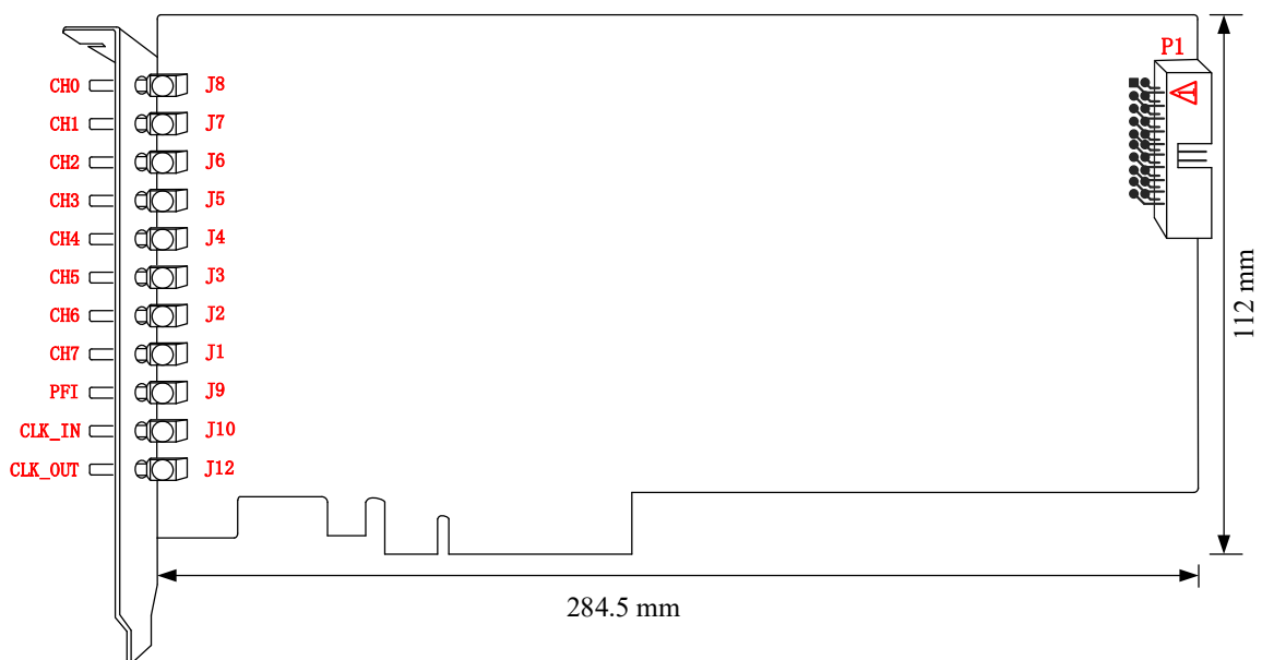
图 3-2-1 PCIe858xA 板卡尺寸图
