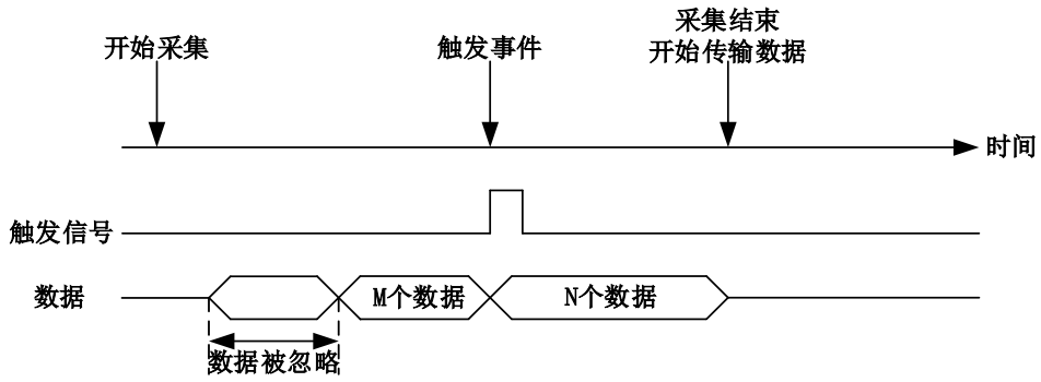
图 4-9-2-2 中间触发
