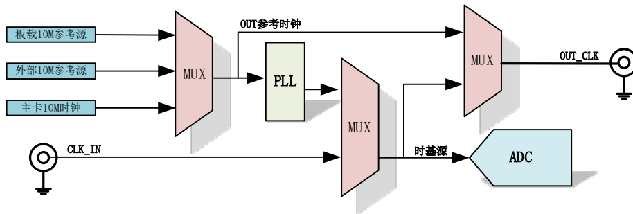
图 4-7-1 时基源框图
