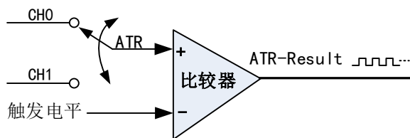
图 4-8-5 比较器
