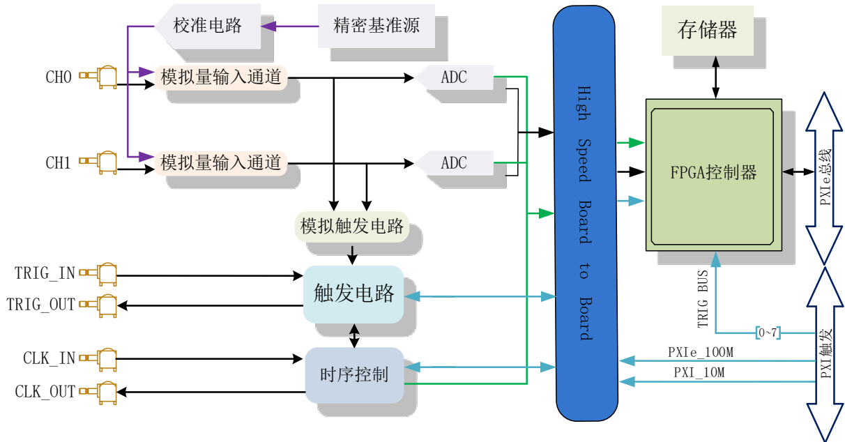
图 3-1-1 PXIe8916A 系统框图
