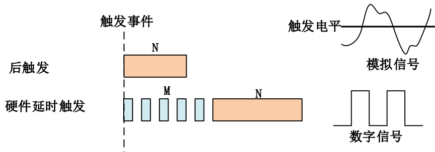
图 4-9-2-1 AD 触发模式
