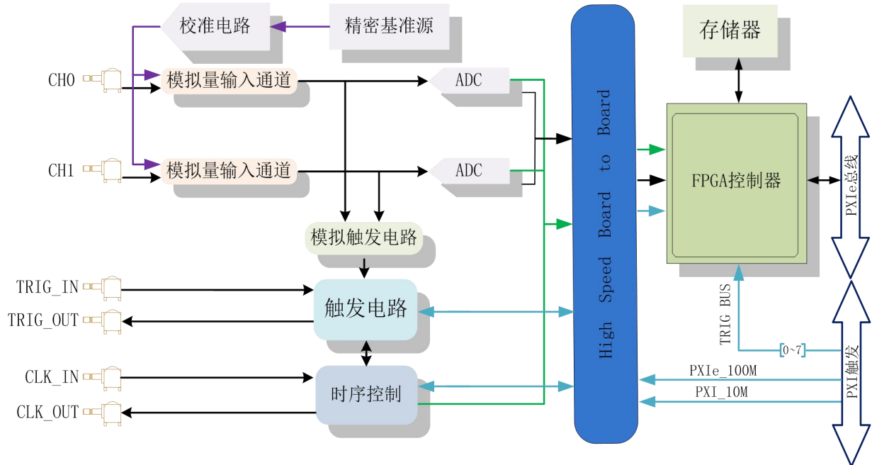
图 3-1-1 PXIe8914A\8912A 系统框图
