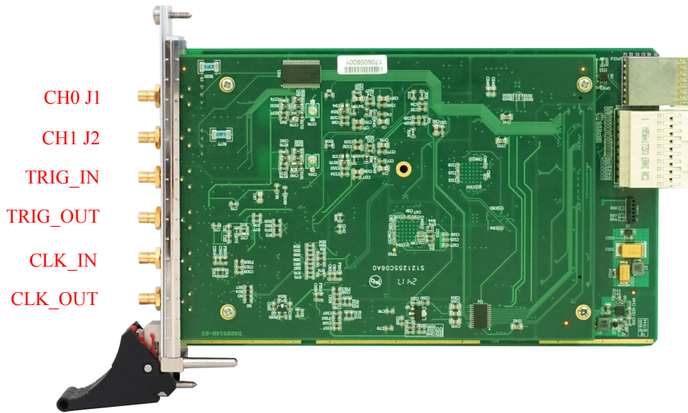
图 3-3-1 PXIe8914A/8912A 产品外观图
