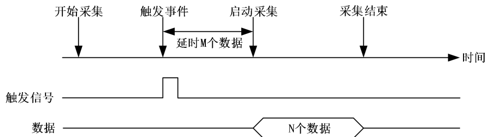
图 4-9-2-3 硬件延时触发
