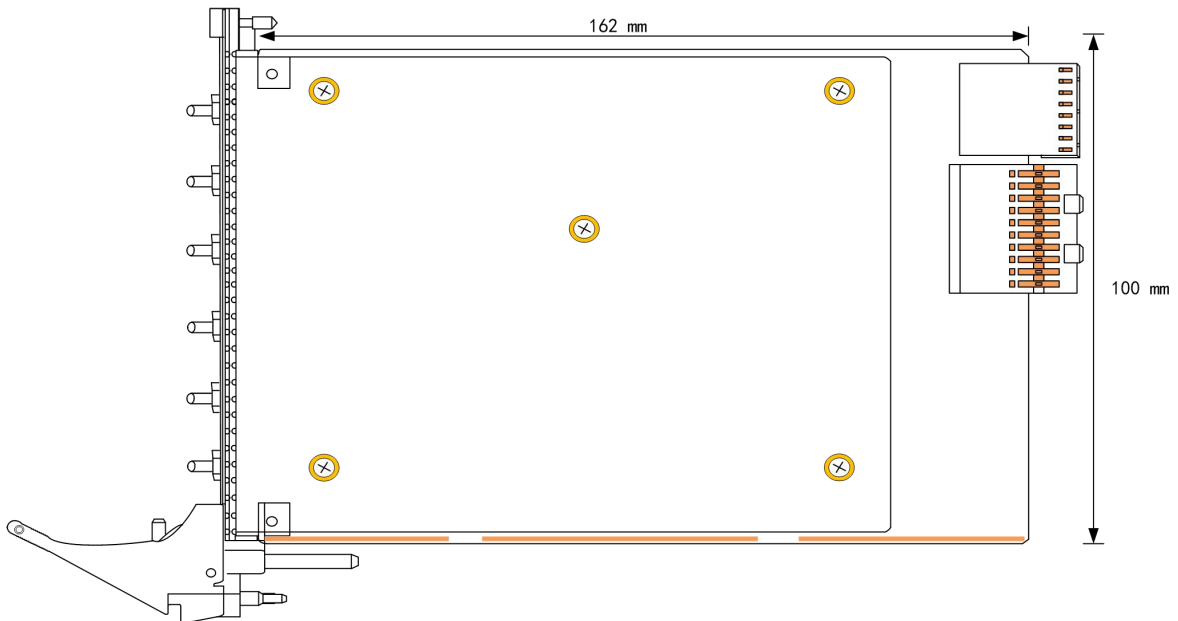
图 3-2-1 PXIe8914A\8912A 板卡尺寸图
