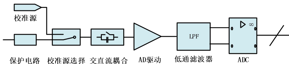
图 4-1-1 AD 功能框图
