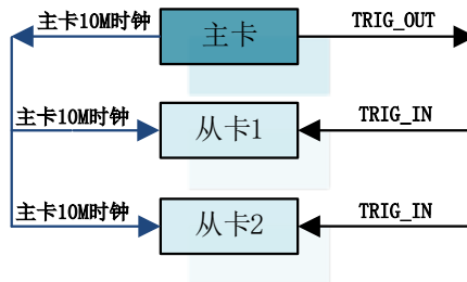
图 4-9-1 主从卡级联
