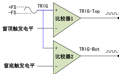
图5-3-4 比较器
