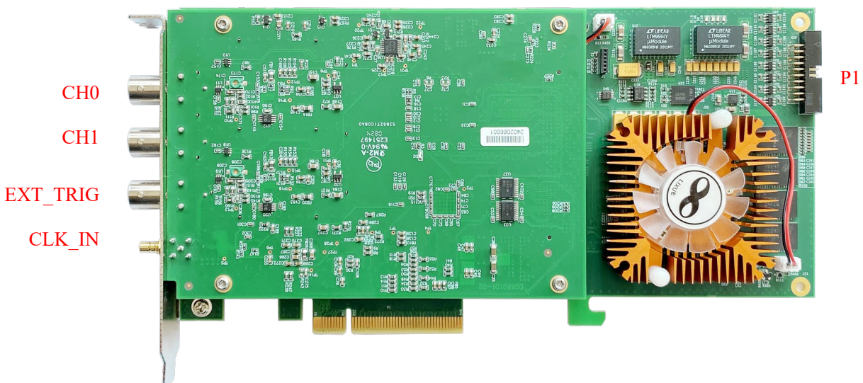
图 3-2-1 PCIe8910N 产品外观图
