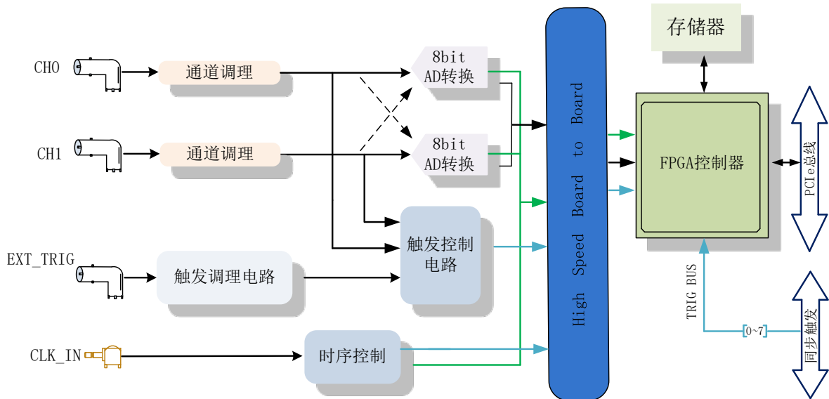
图 3-1-1 PCIe8910N 系统框图
