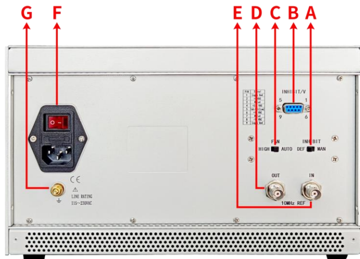
图 3 后面板
