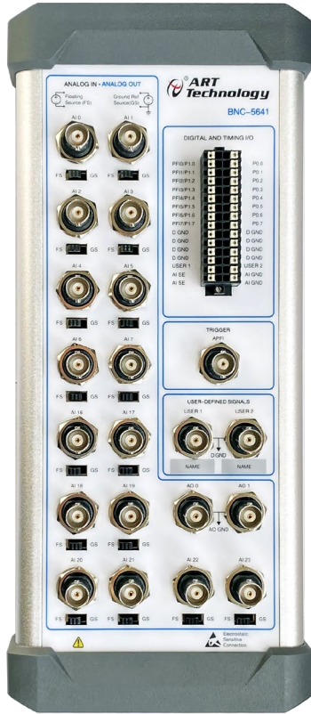
图 3-3-1 BNC-5641 顶视图
