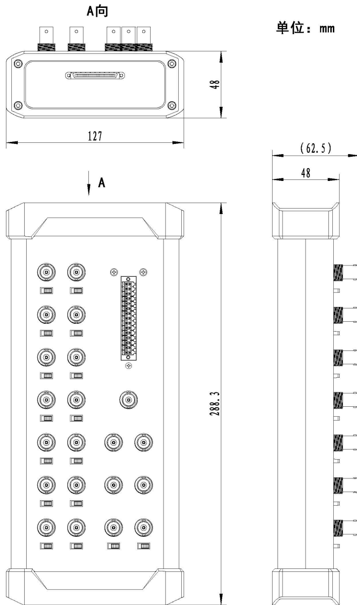
图 3-4-1 BNC-5641 尺寸图
