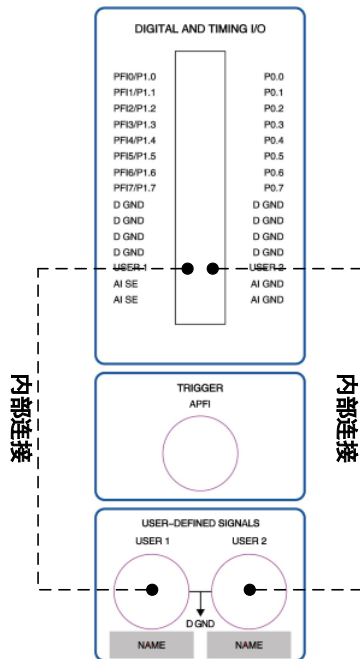
数字和定时 I/O 弹簧端子
