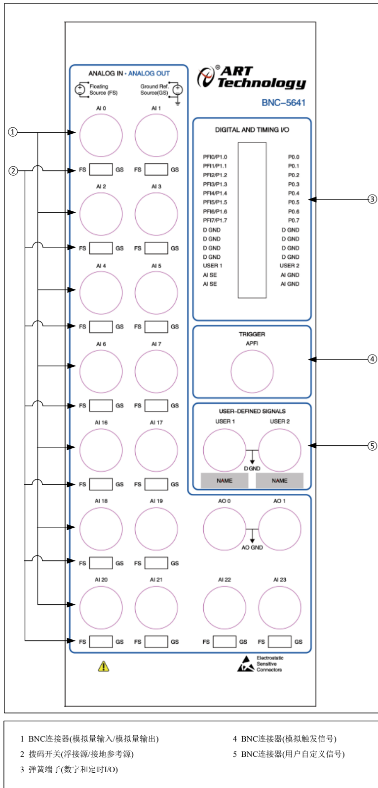
图 2-1 BNC-5641 前面板
