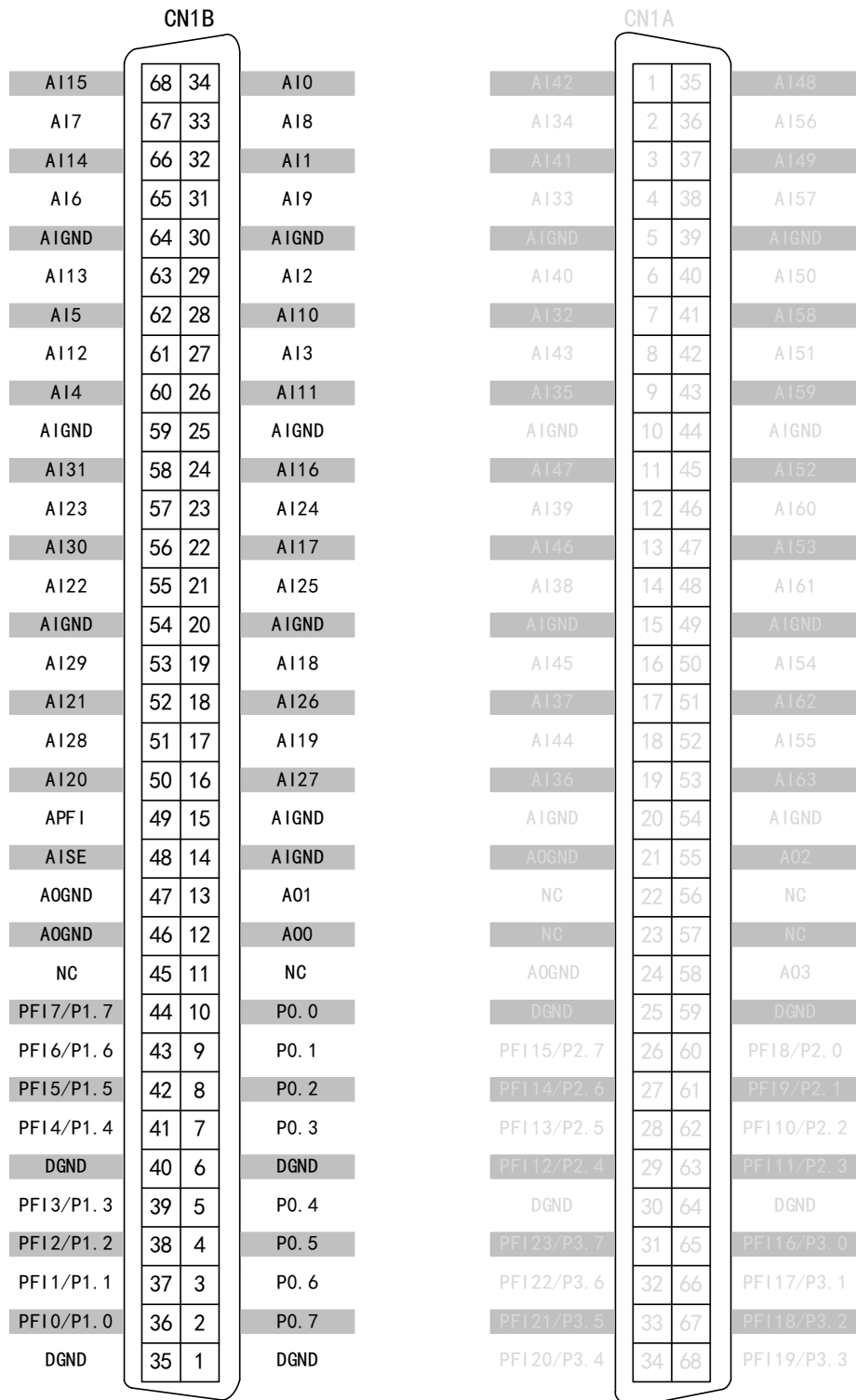
PCI/PCIe 5640/5680 DAQ 设备连接器管脚定义
