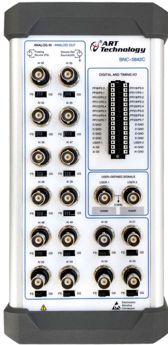
图 3-3-1 BNC-5642C 顶视图
