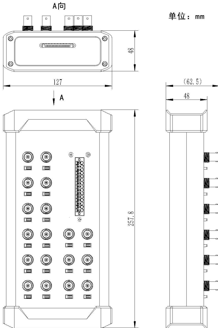
图 3-4-1 BNC-5642C 尺寸图
