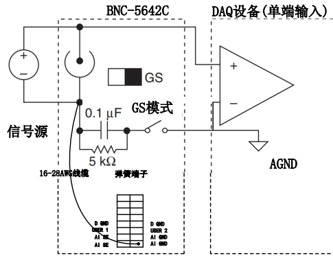
图 4-1-3 测量一个单端模式下的浮接信号
