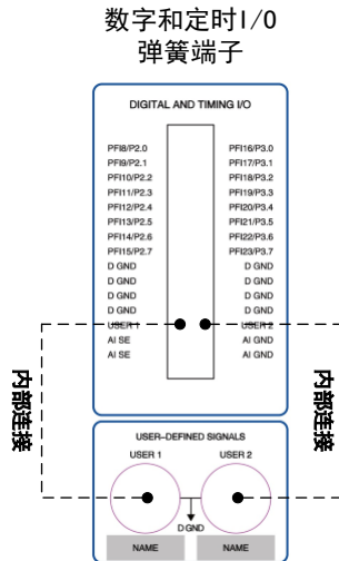
图 4-3-1 USER<1..2>BNC 连接器内部连接
