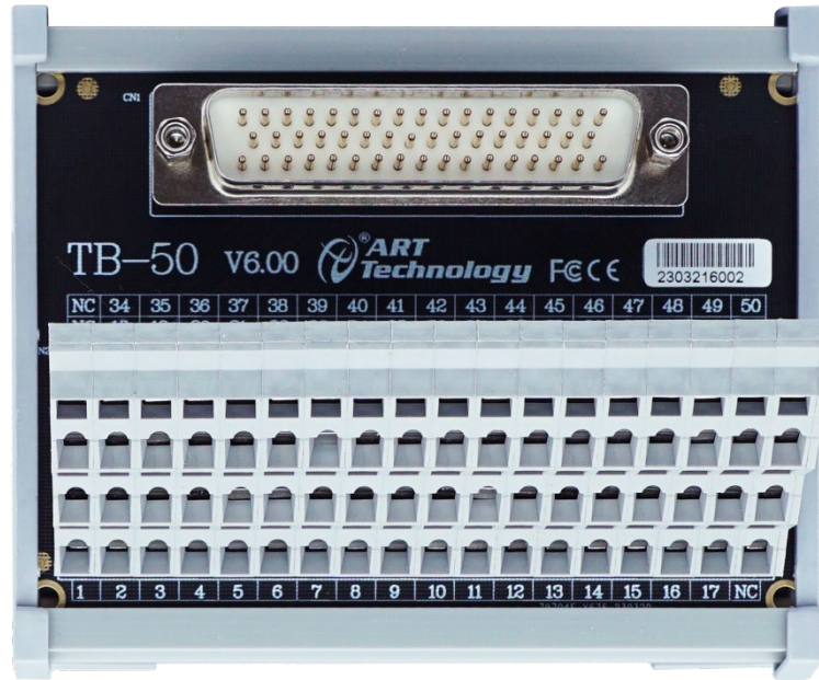
图 1 端子台顶视图
