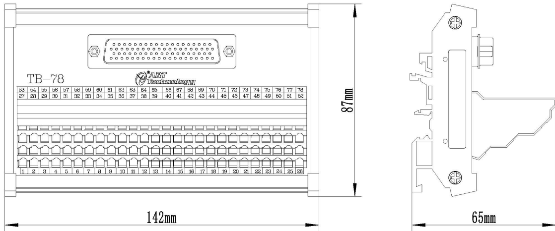
图 3 产品尺寸图
