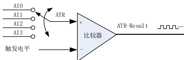
图 4-8-5 比较器
