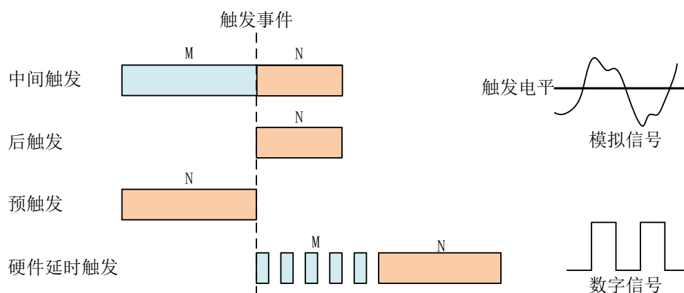
图 4-9-2-1 AI 触发模式
