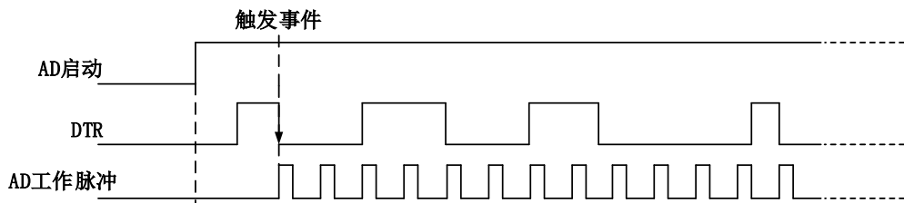
图 4-8-9 DTR 触发--下降沿触发
