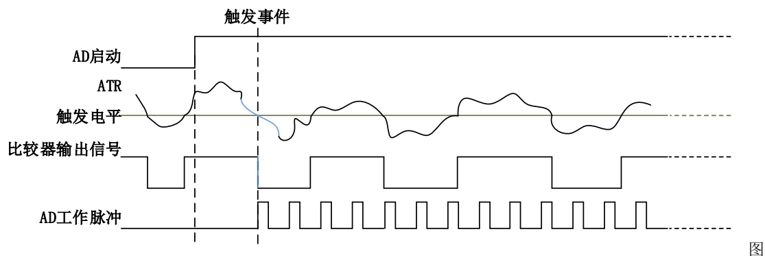
4-8-6 ATR 触发--下降沿触发
