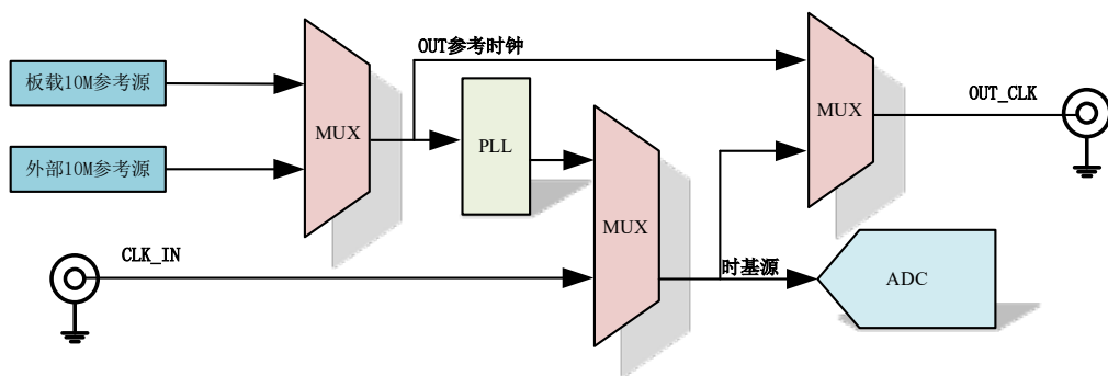
图 4-7-1 时基源框图
