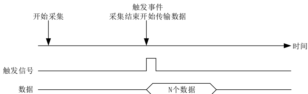
图 4-9-2-3 后触发
