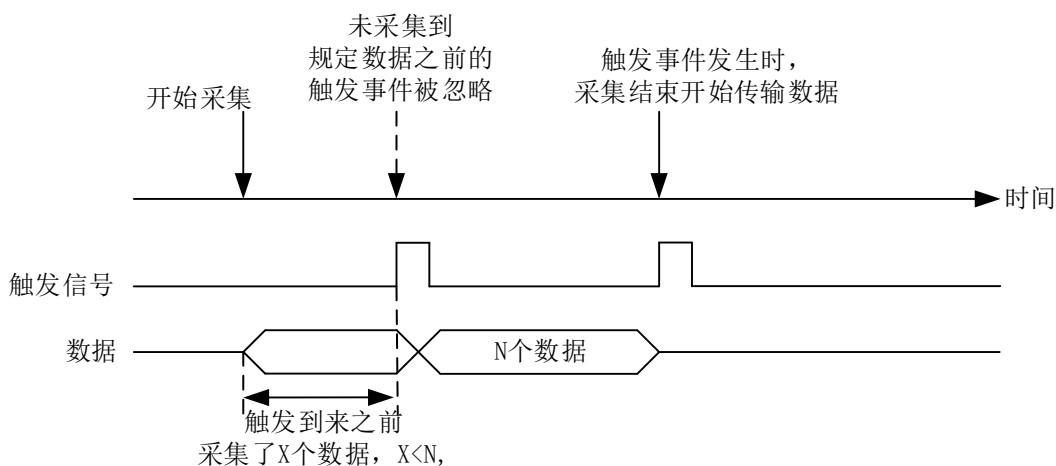
图 4-9-2-5 预触发--采集数据小于 N
