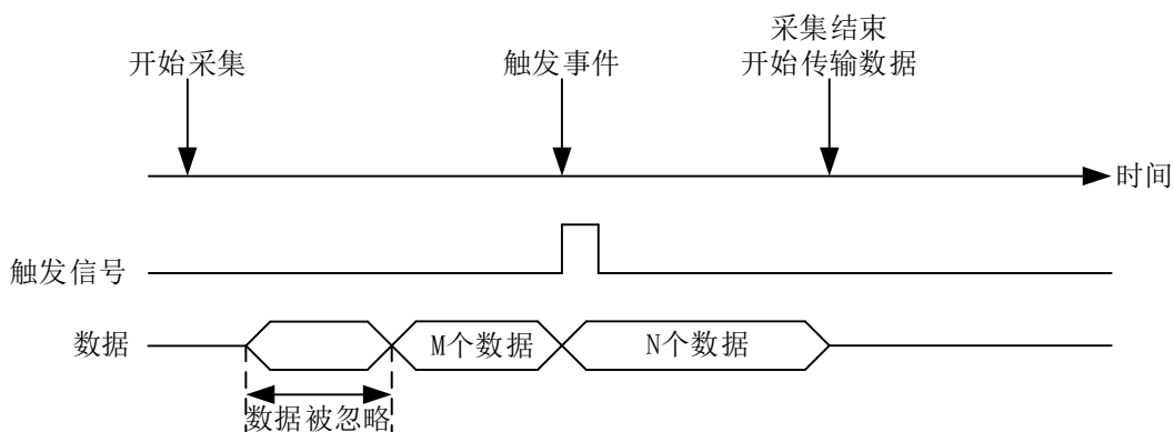
图 4-9-2-2 中间触发
