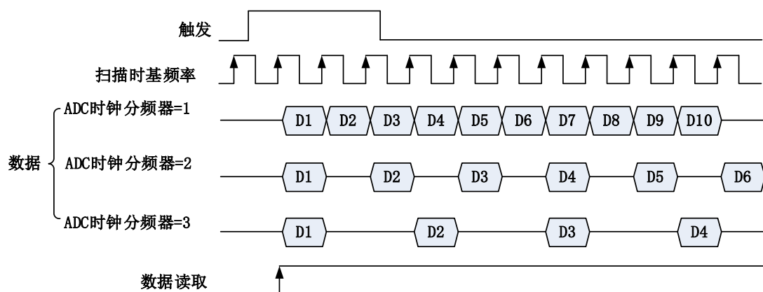
图 4-7-2 AD 抽样速率示意图
