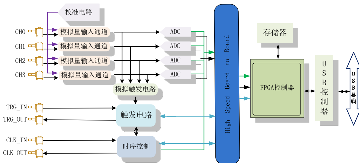
图 3-1-1 USB853x 系统框图
