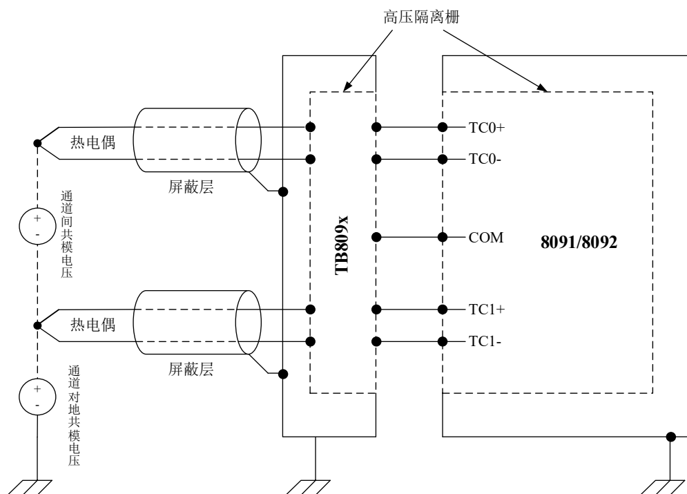
图 4-1-1 外接屏蔽热电偶示意图
