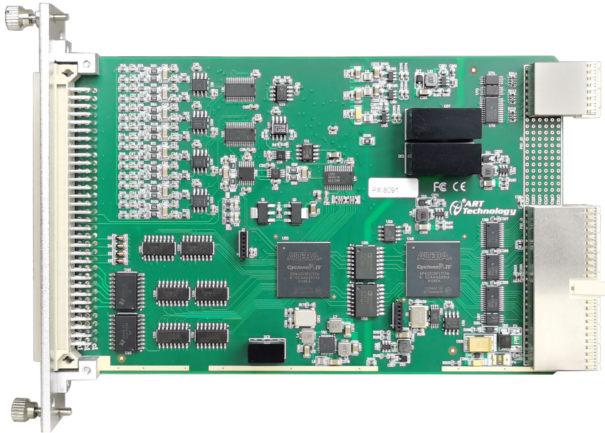
图 3-1-1 PXI8091 外形图
