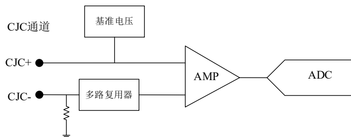
图 4-6-1 冷端补偿示连接意图
