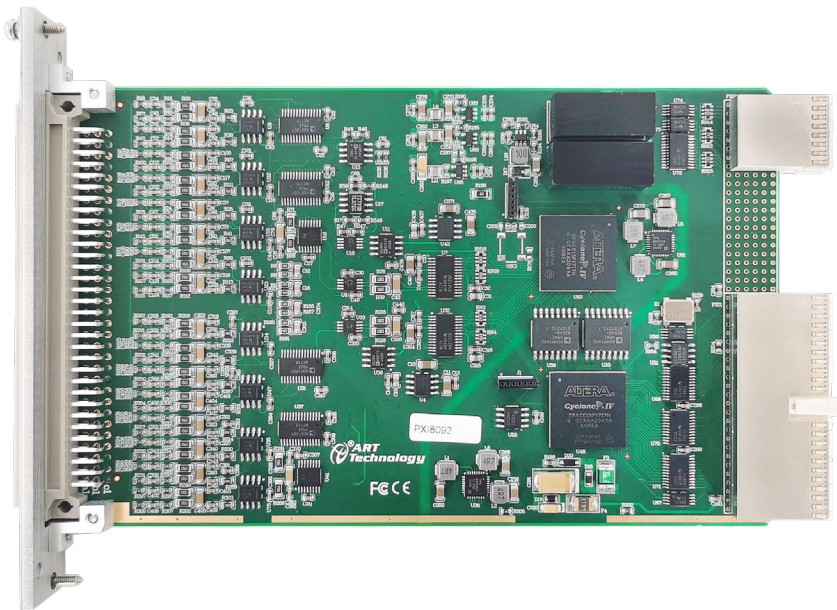
图 3-1-2 PXI8092 外形图
