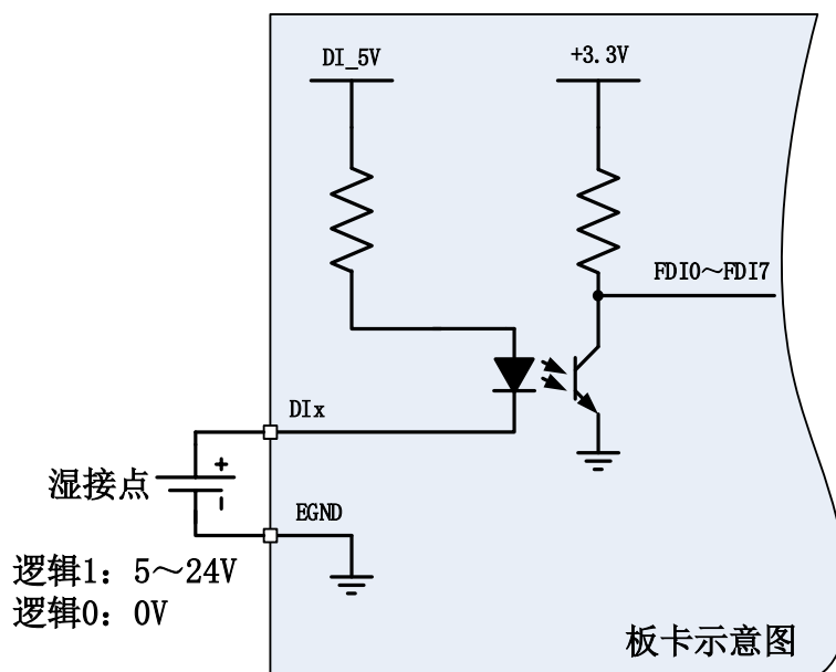
图 5-1-2 湿接点接线方式
