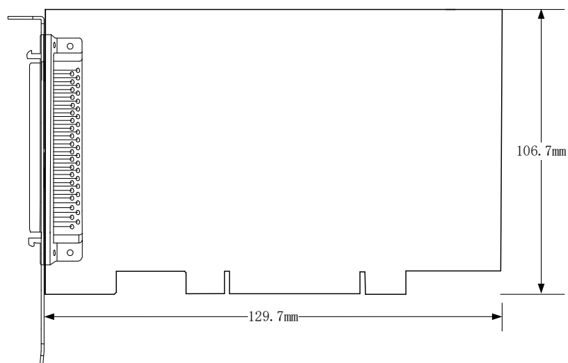
图 3-2-2 PCI2355/2356/2357 结构图
