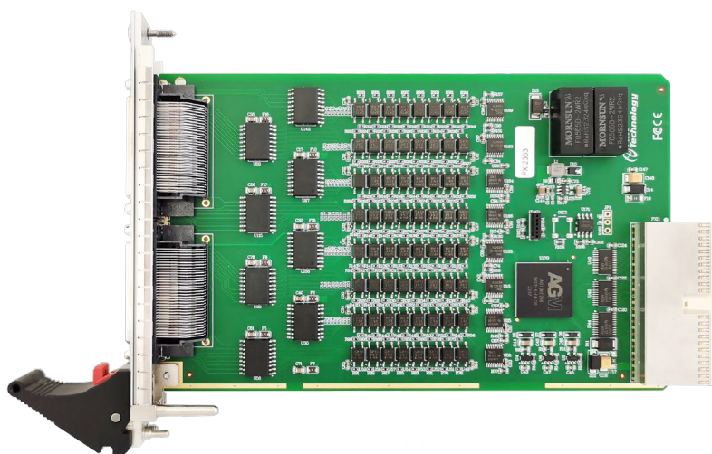
图 3-1-4 PXI2353 外形图
