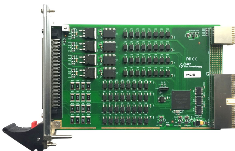
图 3-1-5 PXI2355 外形图
