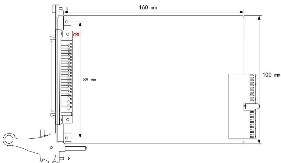
图 3-2-3 PXI2355 结构图
