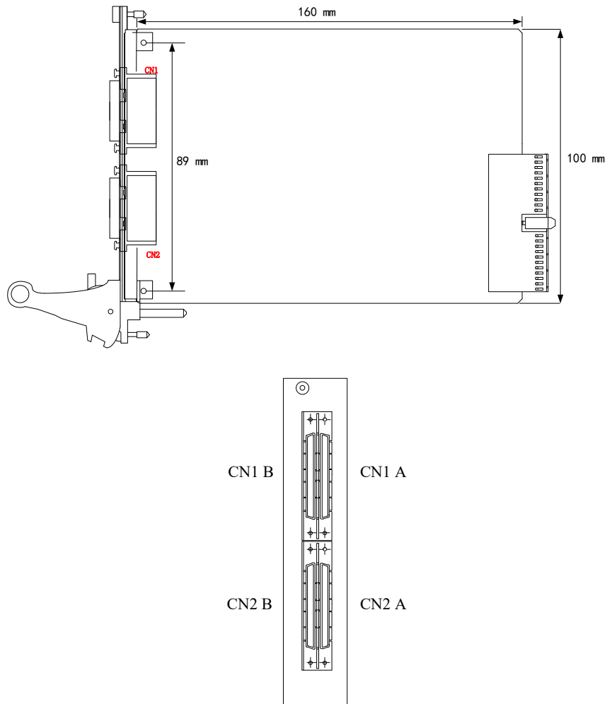
图 3-2-4 PXI2351/PXI2353 结构图及连接器正面示意图
