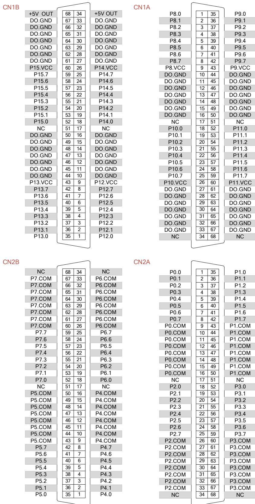
图 3-3-1 PCI2351/PXI2351 接口定义
