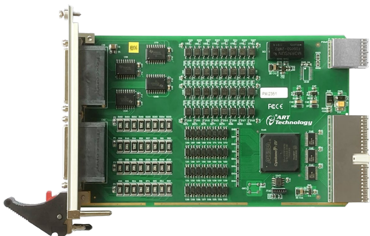
图 3-1-3 PXI2351 外形图
