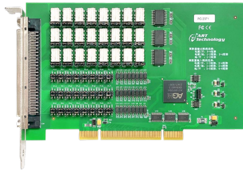
图 3-1-7 PCI2371 外形图
