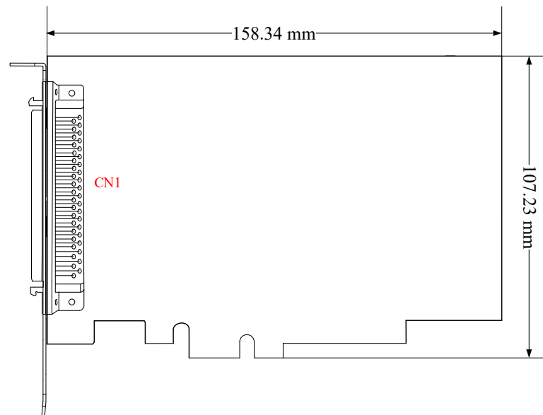
图 3-2-3 PCIe237x 尺寸图
