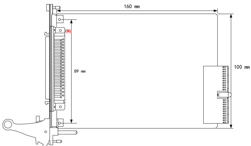
图 3-2-1 PXI237x、CPCI237x 尺寸图
