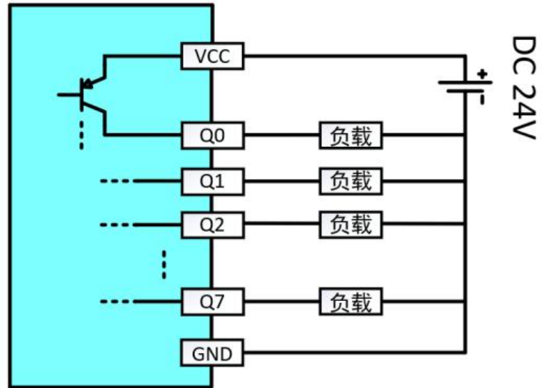
图3 输出接线
