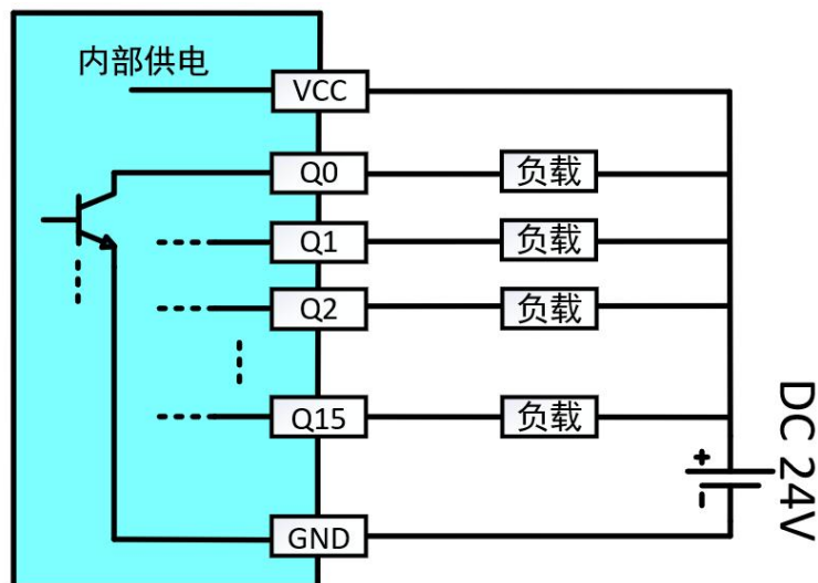
图 2 输出接线
