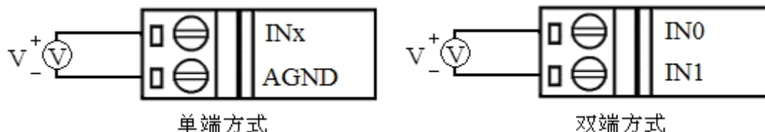
模拟量输入接线图
