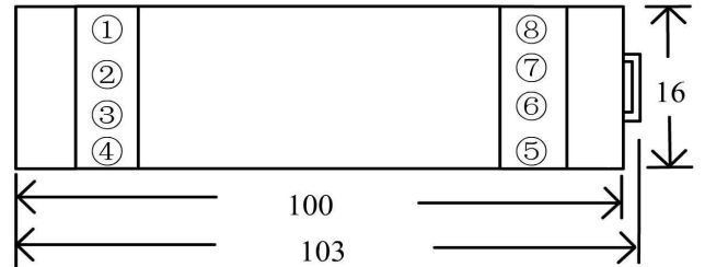
俯视图
