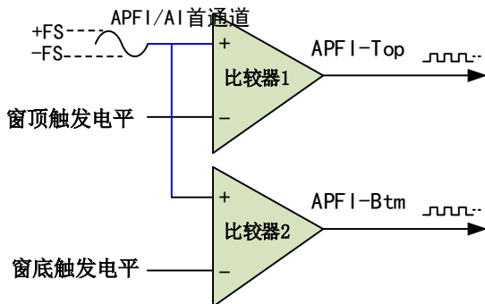
图8-3-6 比较器
