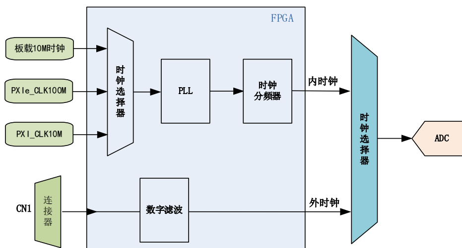
图 4-6-1 975x AI 时钟结构框图
