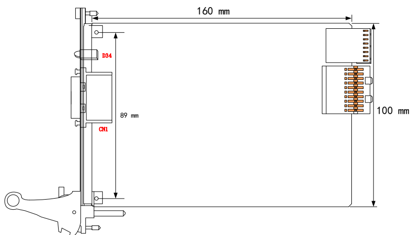
图 3-2-1 PXIe975x (A_B)板卡尺寸图
