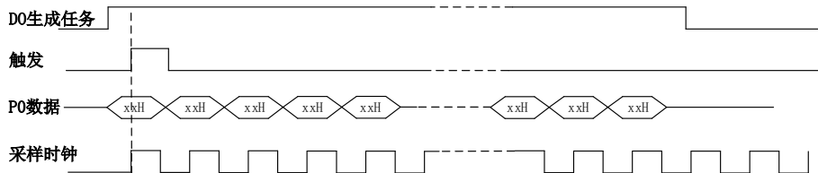
图7-6-3 内、外时钟连续生成
