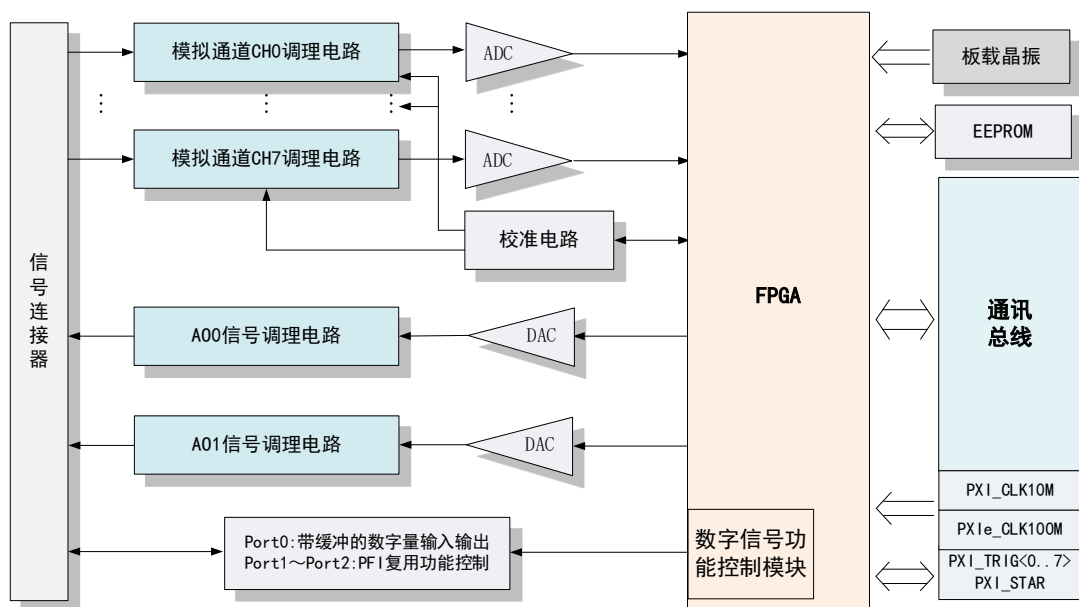
图2-2-1 975x系统框图
