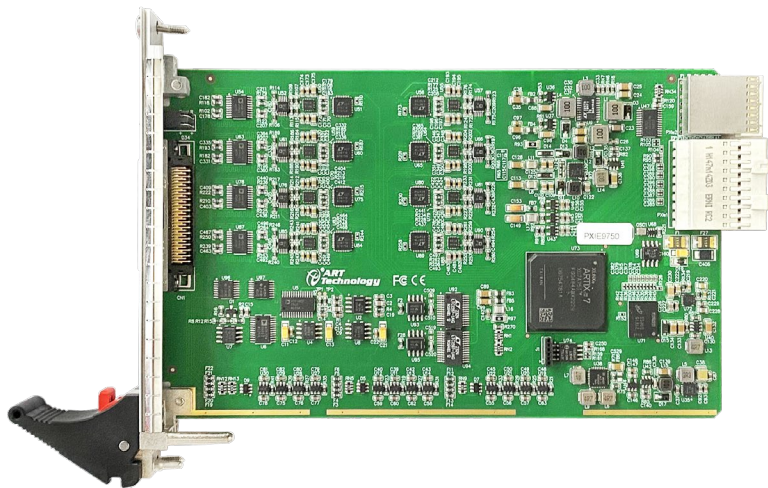
图 3-1-1 PXIe975x (A_B)外观图
