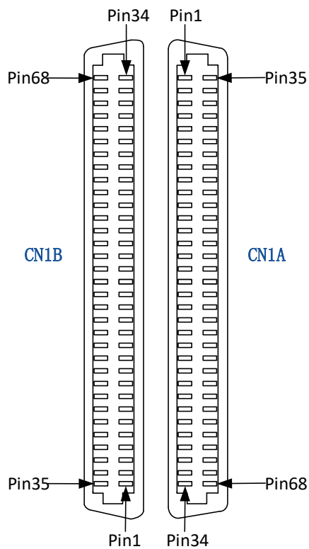
图 3-3-2 CN1 VHDCI 连接器管脚定义
