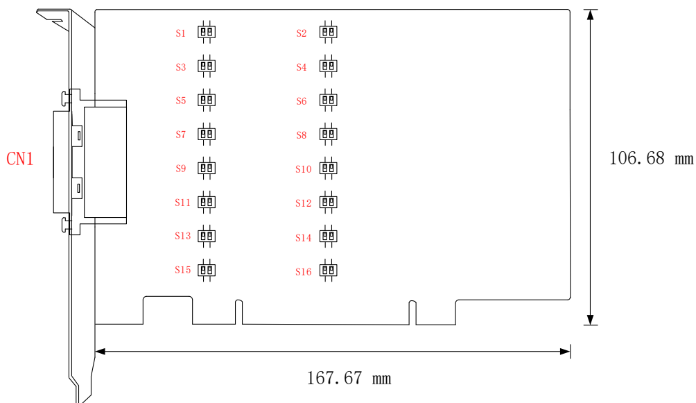
图 3-2-1 板卡尺寸图
