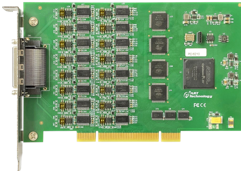
图 3-1-1 PCI6210 外形图
