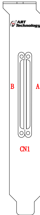
图 3-3-1 连接器正面示意图
