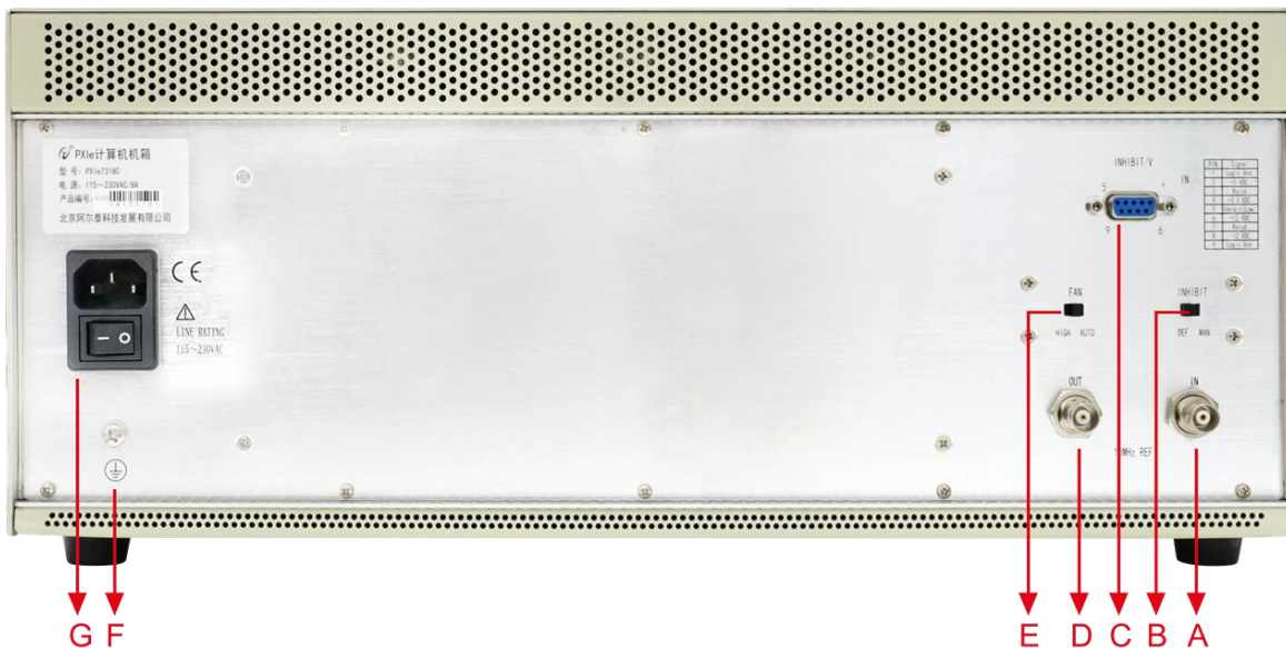
PXIeC-7314-21C 后面板
